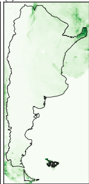
(e) MODIS v6.1 2003
