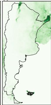
(f) MODIS v6.1 2023
