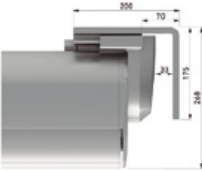
Detalle sujeción entre paredes
