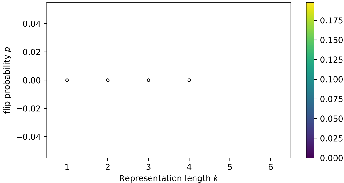
mean branching entropy (subsample=1)
