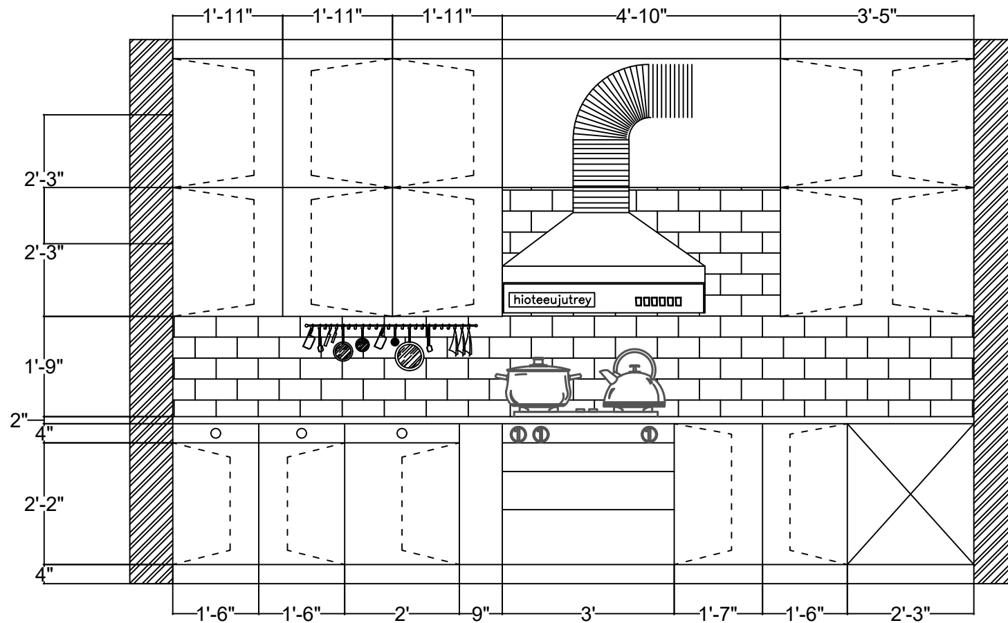
Elevation A
