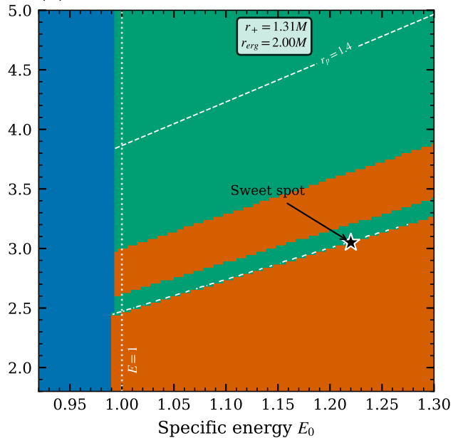
(b) a/M=0.95
