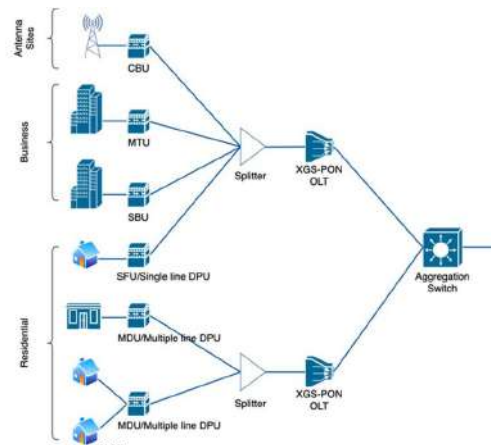
Gambar 3. 21 Jaringan XGS-PON
