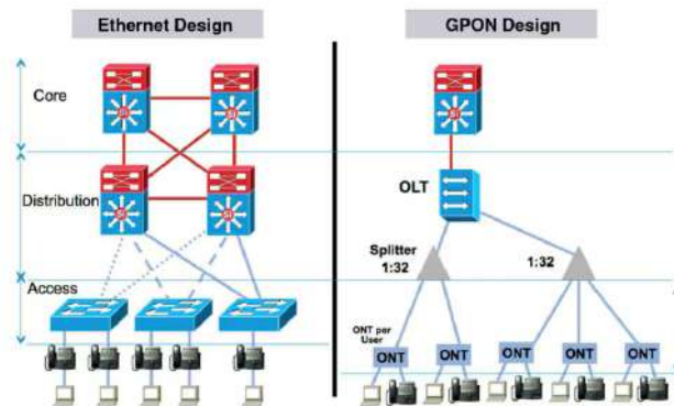
Gambar 3. 19 Perbandingan Desain Ethernet dan GPON
