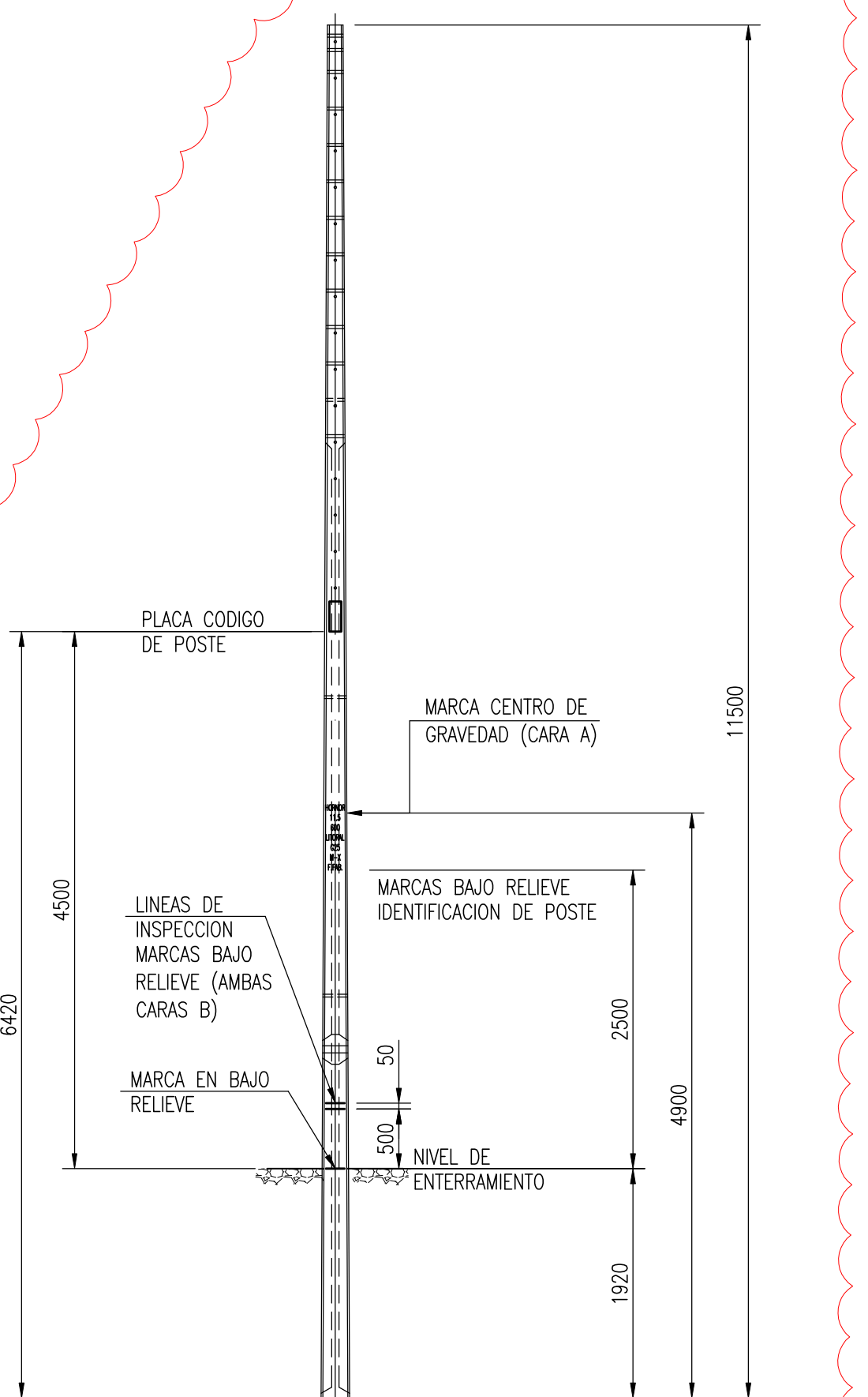
MARCADO DEL POSTE (CARA B) Escala 1:50
