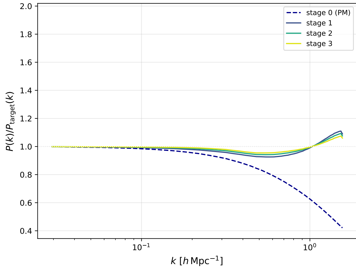
lr = 0.10
