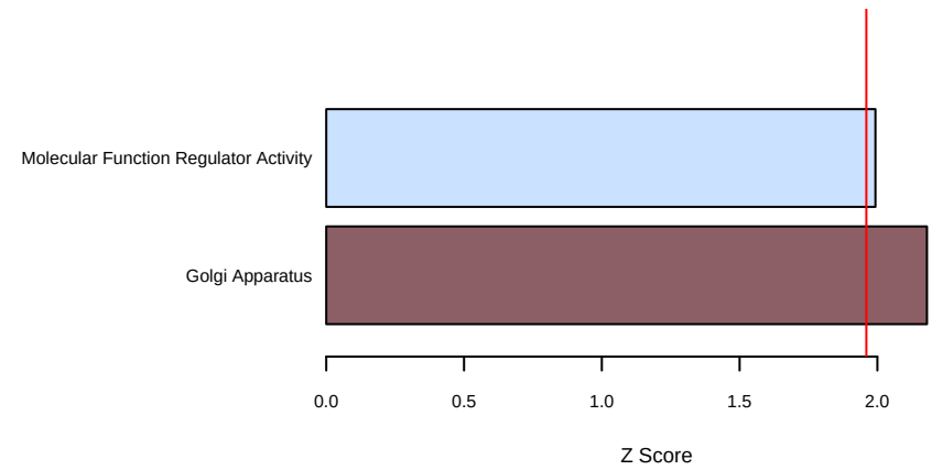
M23 darkturquoise
