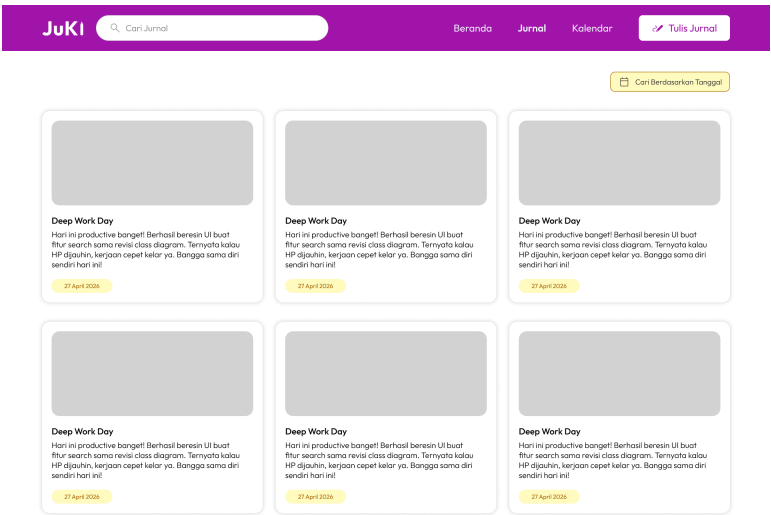
Gambar 3.10 Antarmuka Jurnal
