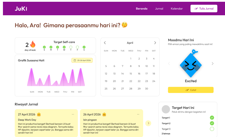
Gambar 3.9 Antarmuka Beranda
