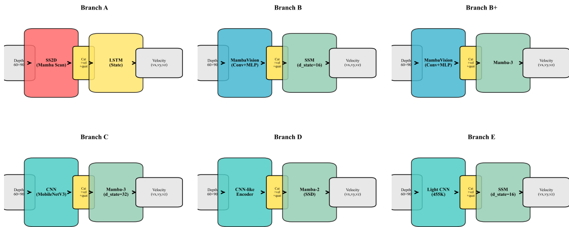
Figure 3.1: 六种 Mamba 学生架构图（从左到右，从上到下：A E）。每个架构图展示了深度图输入、视觉编码器、特征拼接（+ 速度 + 四元数）、时序头和速度输出的完整数据流。彩色编码器区域表示不同类型（SS2D、MambaVision 混合、CNN）。
