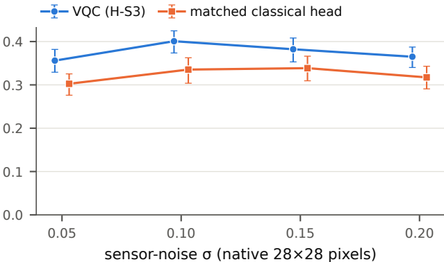
(a) relative F1 loss – relative AUC loss
