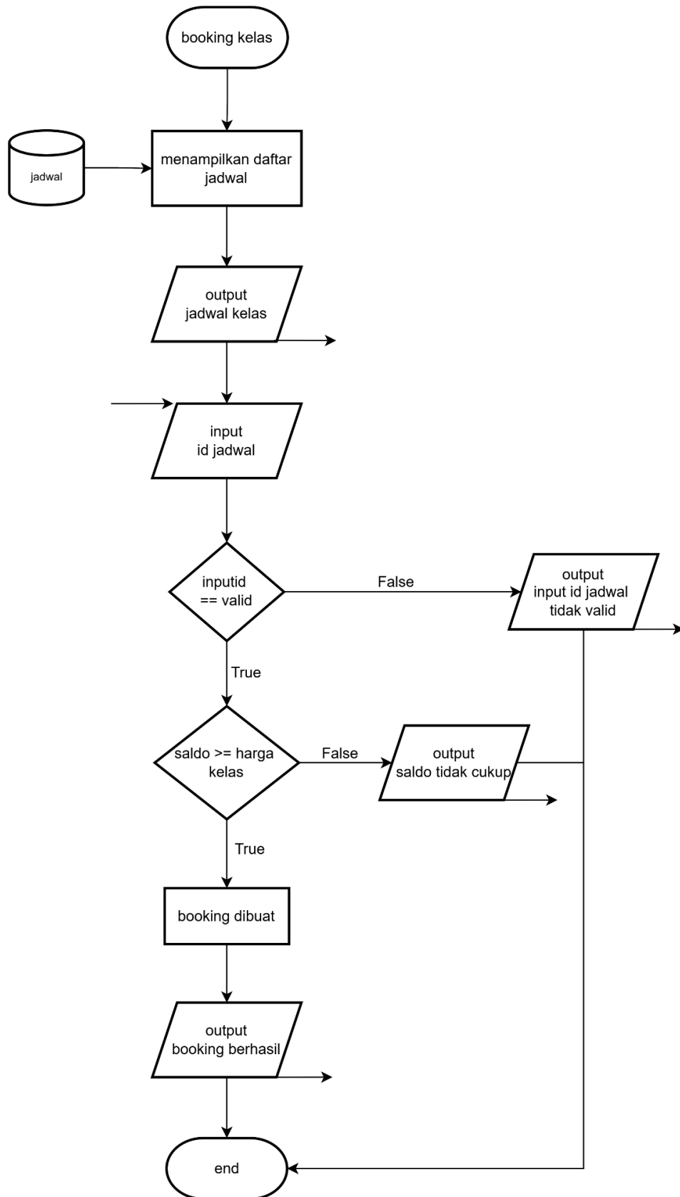
Gambar 2.17 Flowchart Fungsi Booking Kelas Pada Bagian Menu User
