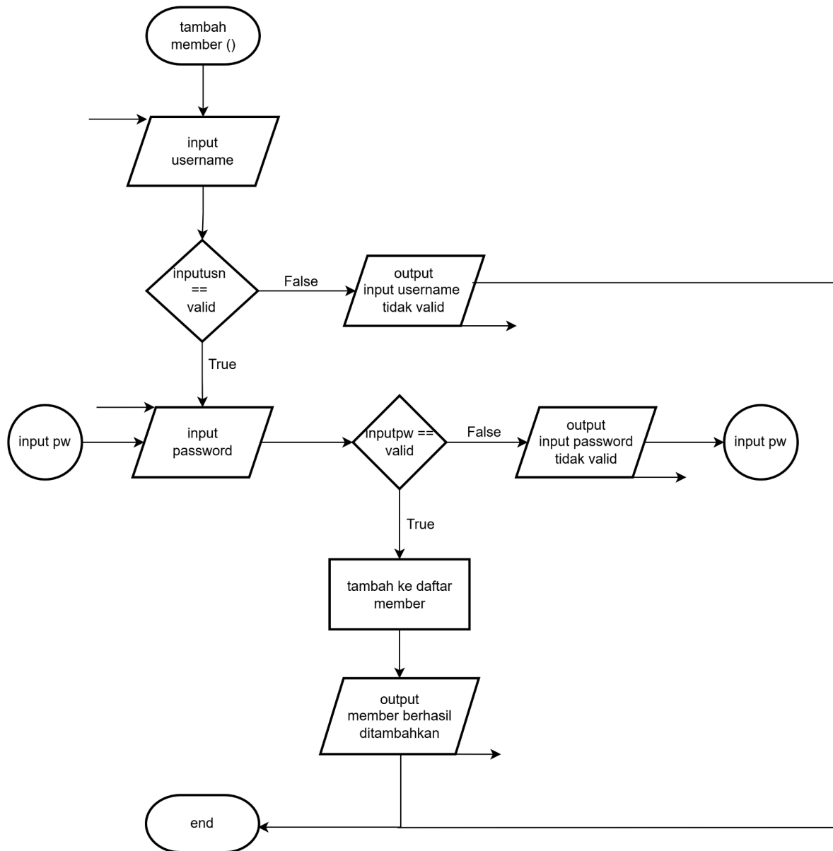
Gambar 2.5 Flowchart Fungsi Tambah Member Pada Bagian Menu Admin
