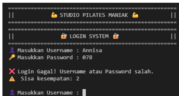
Gambar 3.5 Menu Login (login gagal username salah)
