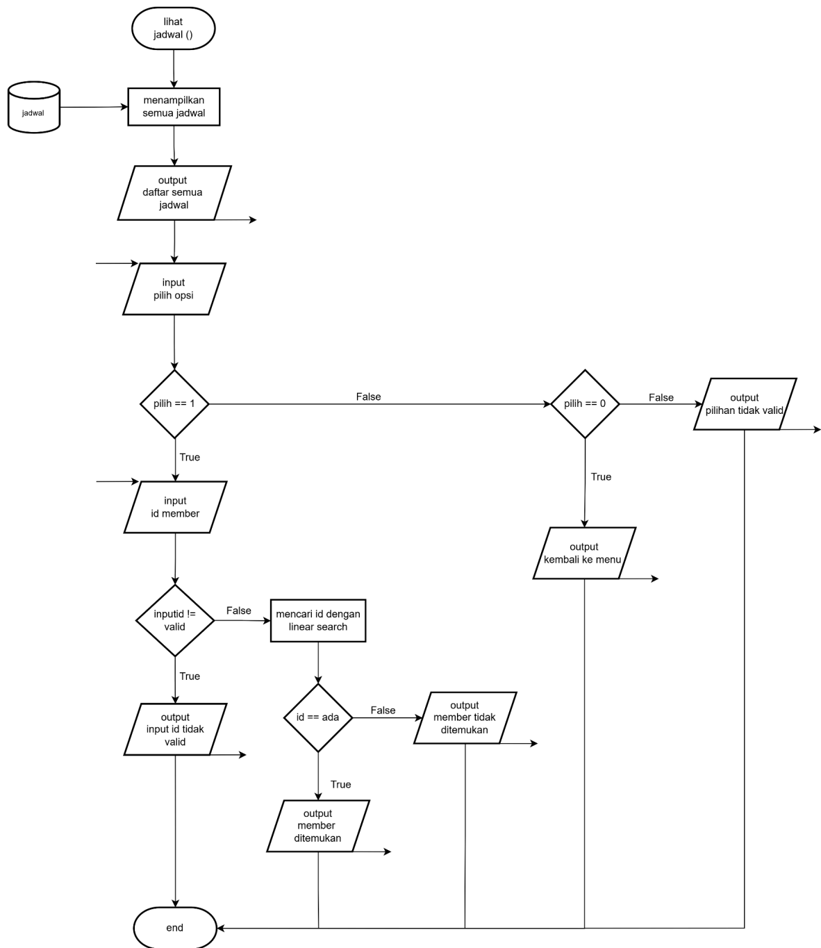
Gambar 2.9 Flowchart Fungsi Lihat Jadwal Pada Bagian Menu Admin
