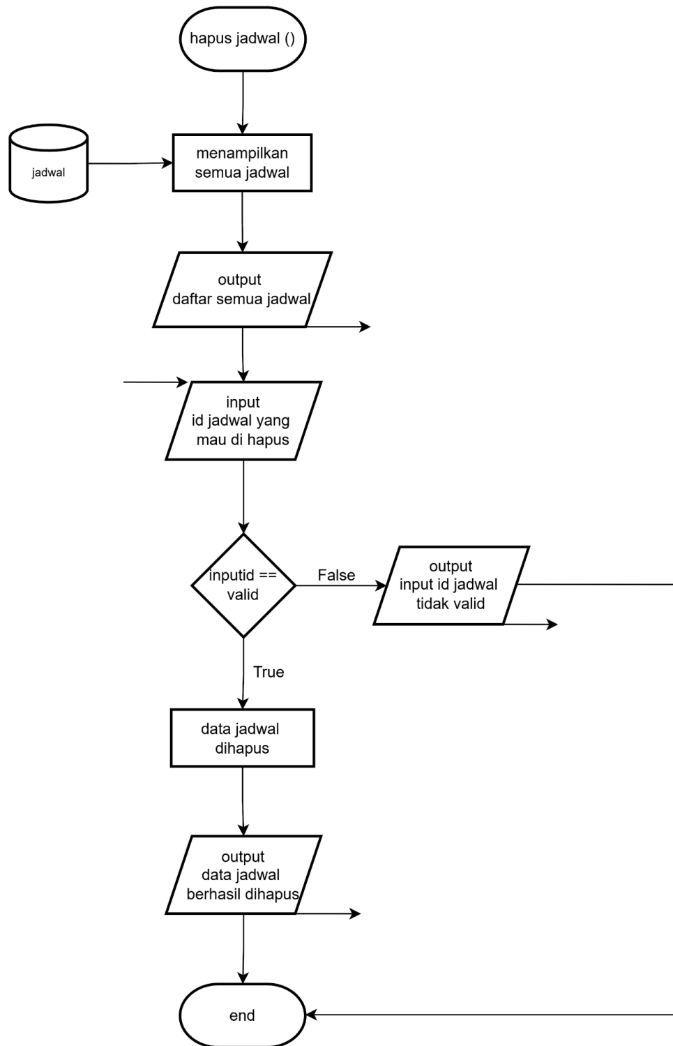
Gambar 2.12 Flowchart Fungsi Hapus Jadwal Pada Bagian Menu Admin
