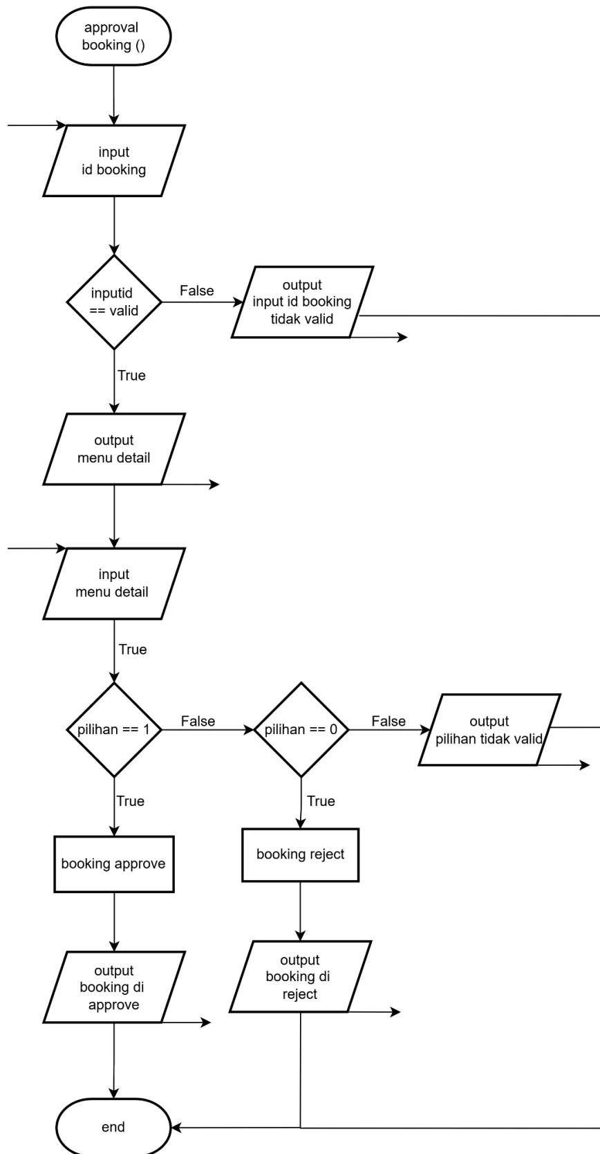
Gambar 2.13 Flowchart Fungsi Approval Booking Pada Bagian Menu Admin
