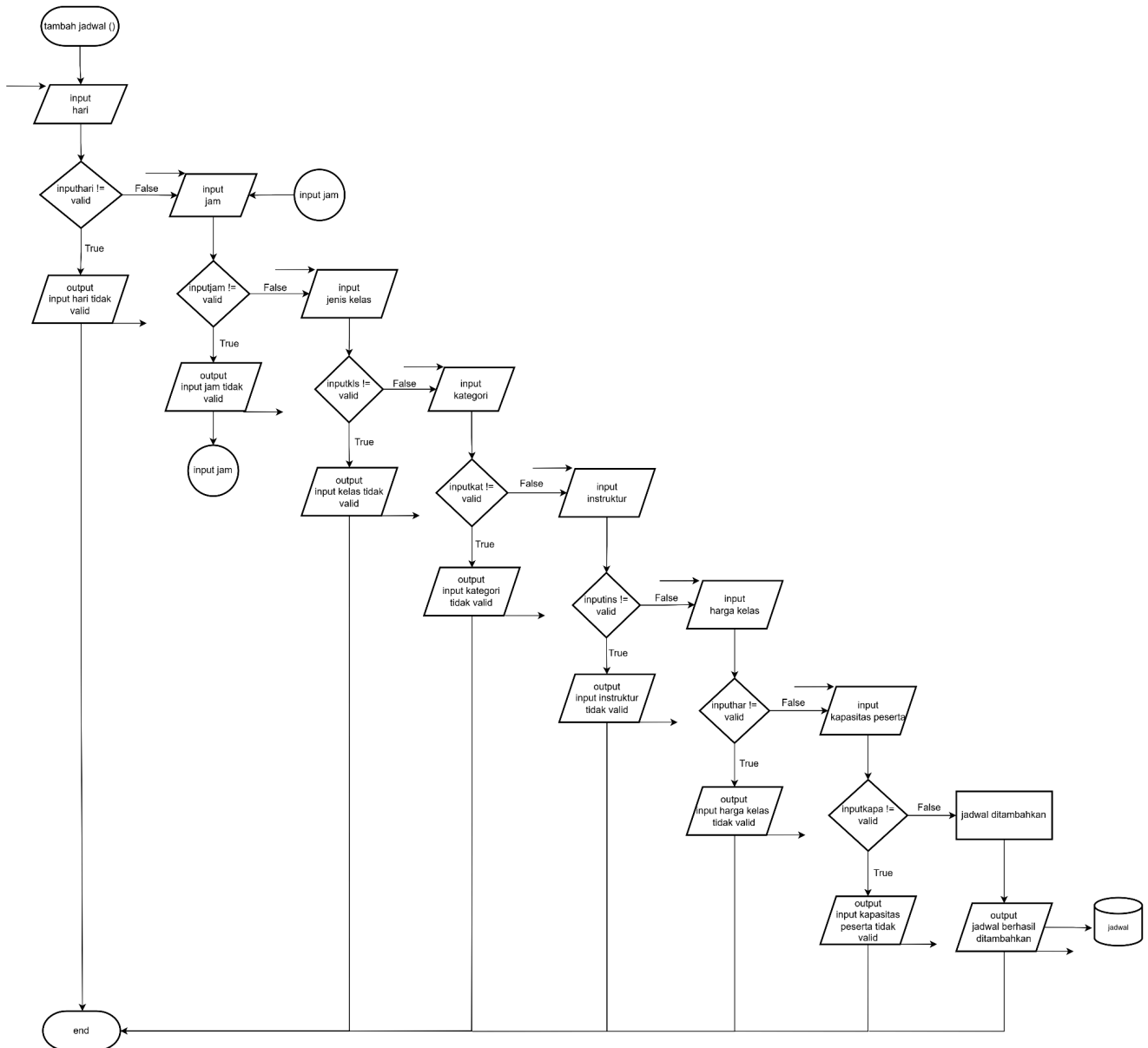
Gambar 2.8 Flowchart Fungsi Tambah Jadwal Pada Bagian Menu Admin
