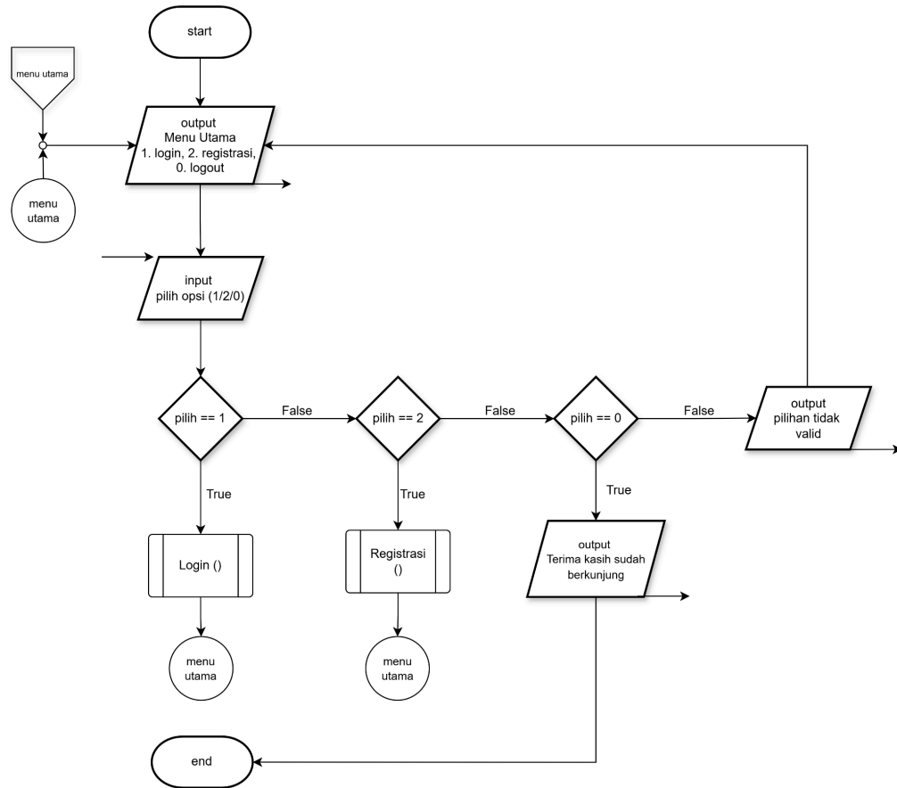
Gambar 2.1 Flowchart Menu Utama
