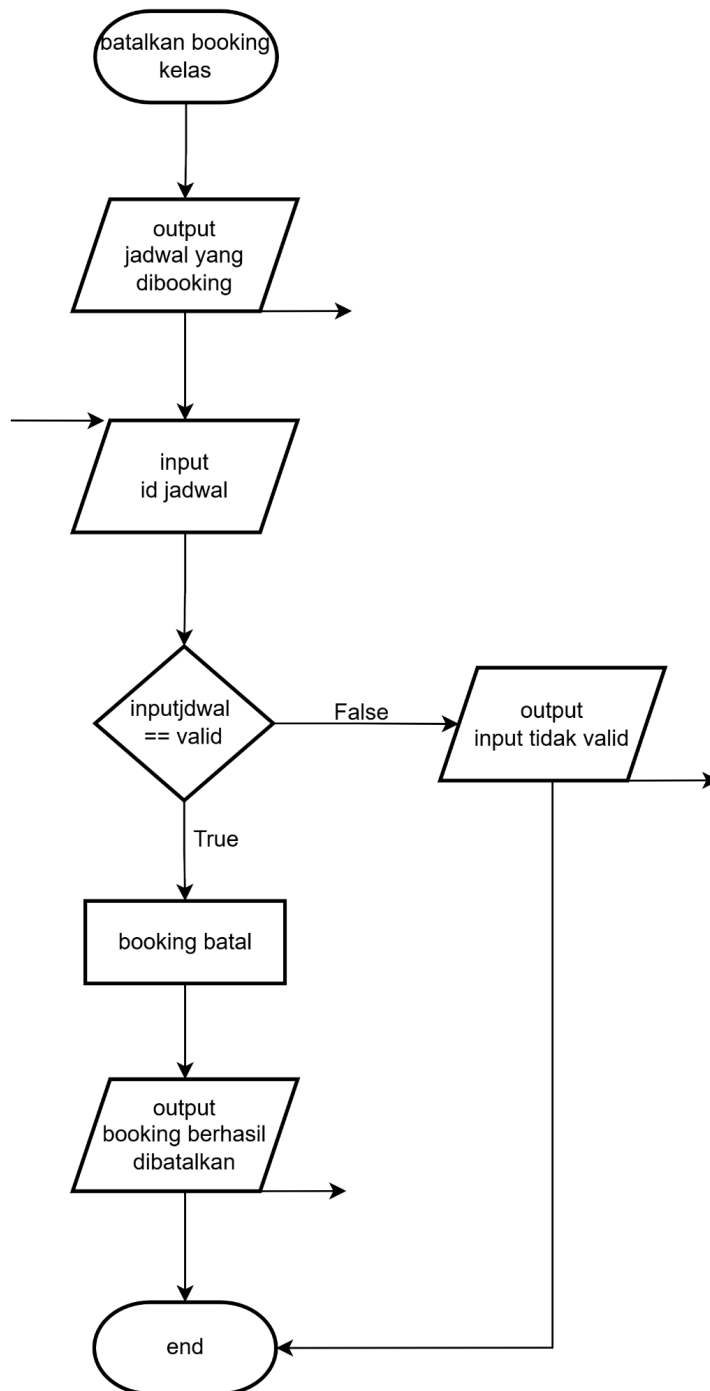
Gambar 2.18 Flowchart Fungsi Batalkan Booking Kelas Pada Bagian Menu User
