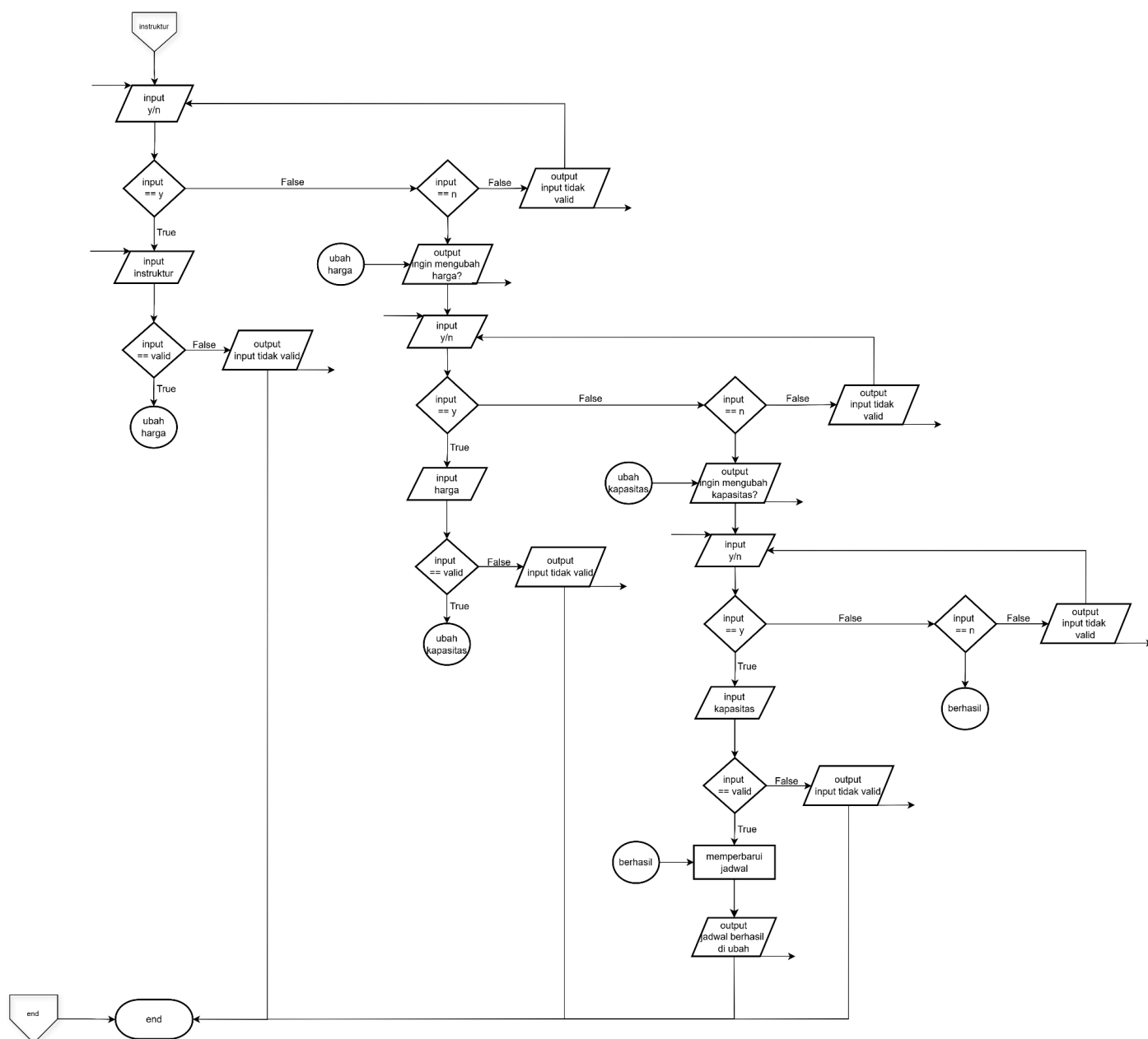
Gambar 2.11 Flowchart Fungsi Update Jadwal 2 Pada Bagian Menu Admin
