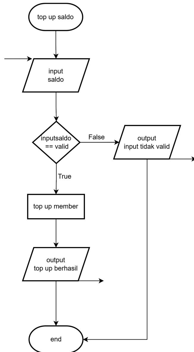
Gambar 2.16 Flowchart Fungsi Top Up Saldo Pada Bagian Menu Admin
