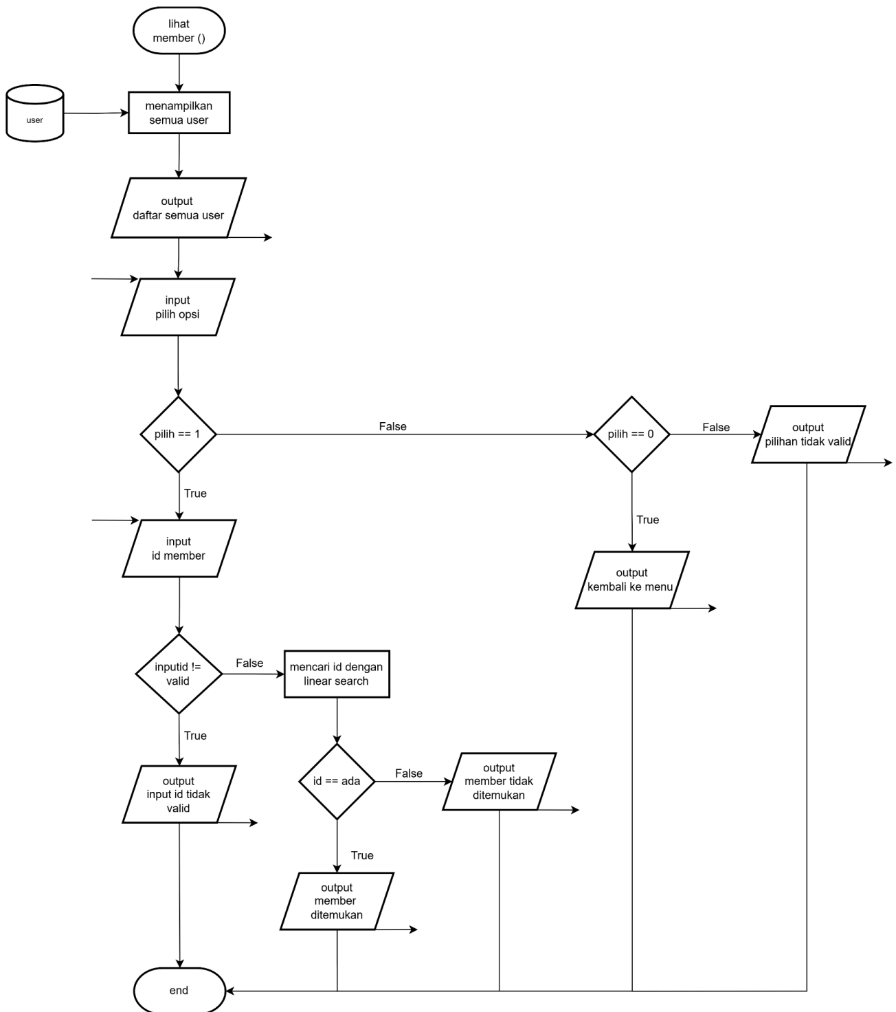
Gambar 2.6 Flowchart Fungsi Lihat Member Pada Bagian Menu Admin
