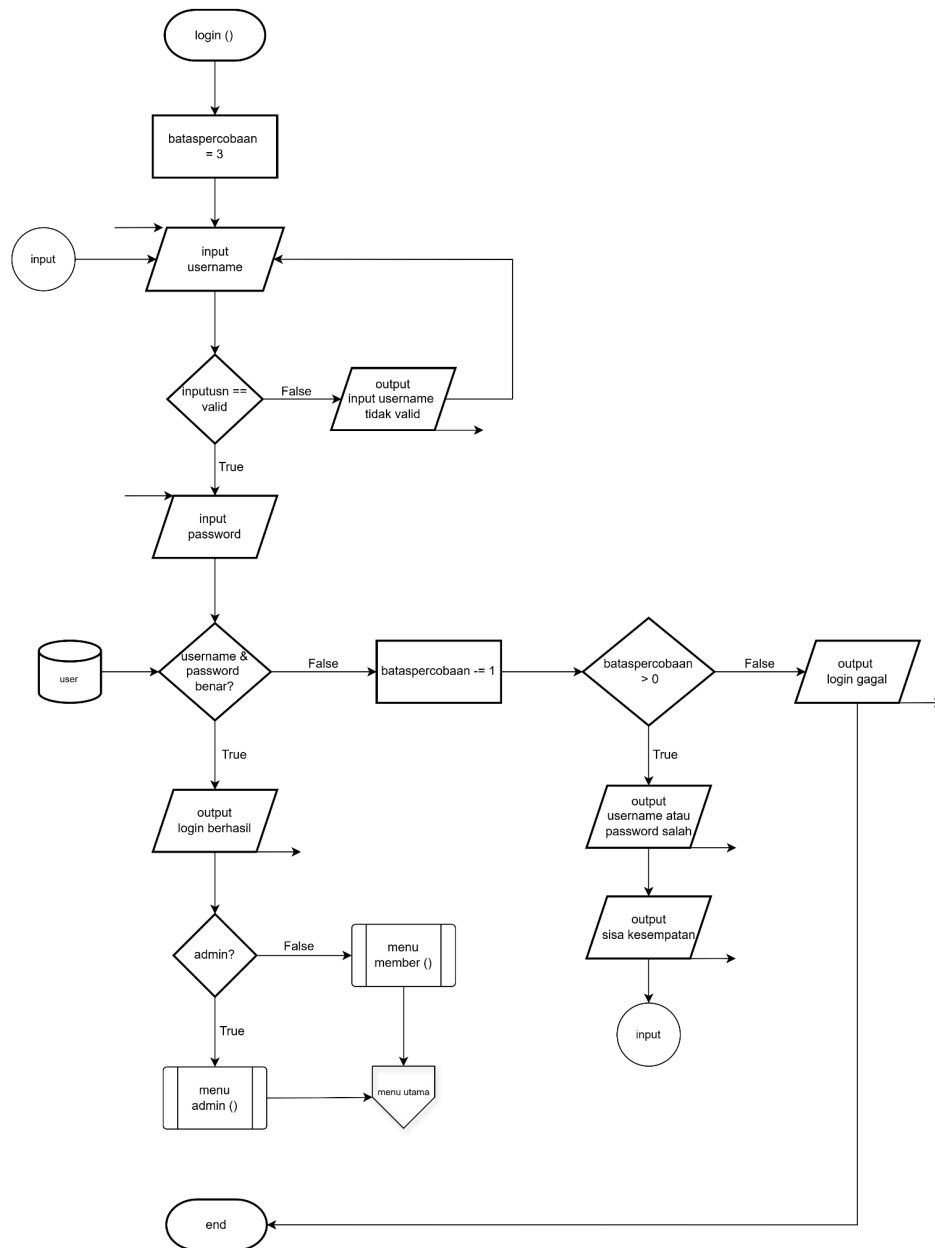
Gambar 2.2 Flowchart Fungsi Login Pada Bagian Menu Utama
