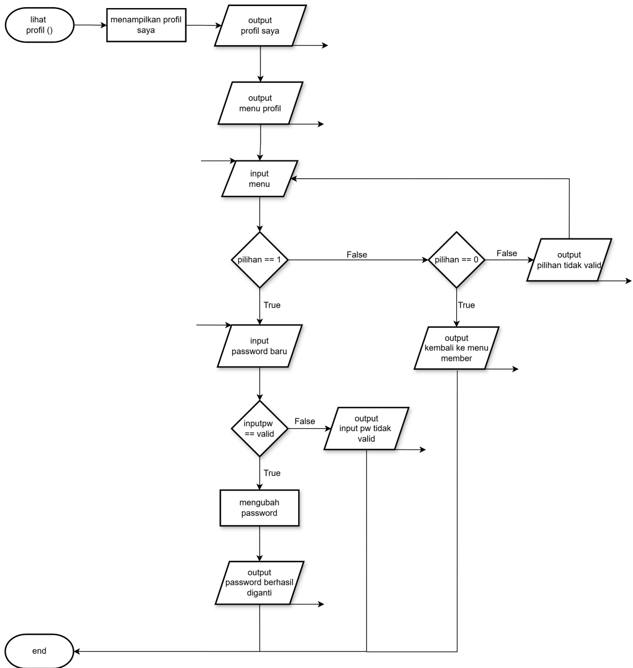
Gambar 2.15 Flowchart Fungsi Profil Pada Bagian Menu User
