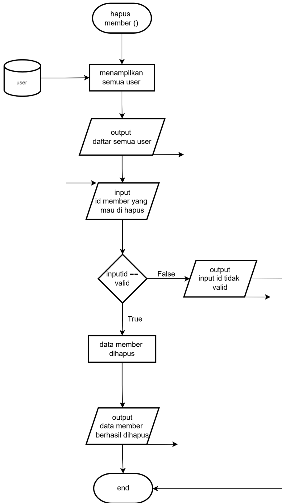
Gambar 2.7 Flowchart Fungsi Hapus Member Pada Bagian Menu Admin
