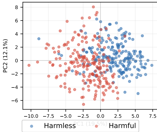
KD-Chat Layer 2
