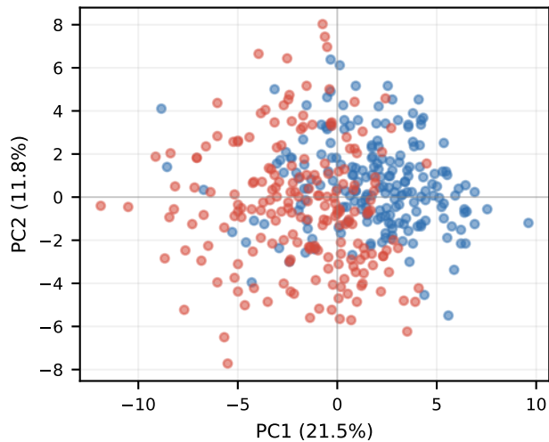
Base Layer 2
