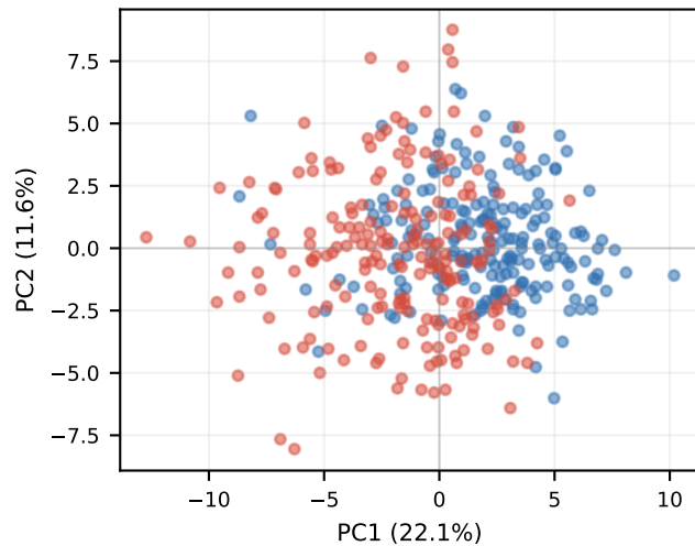
KD-NonChat Layer 2
