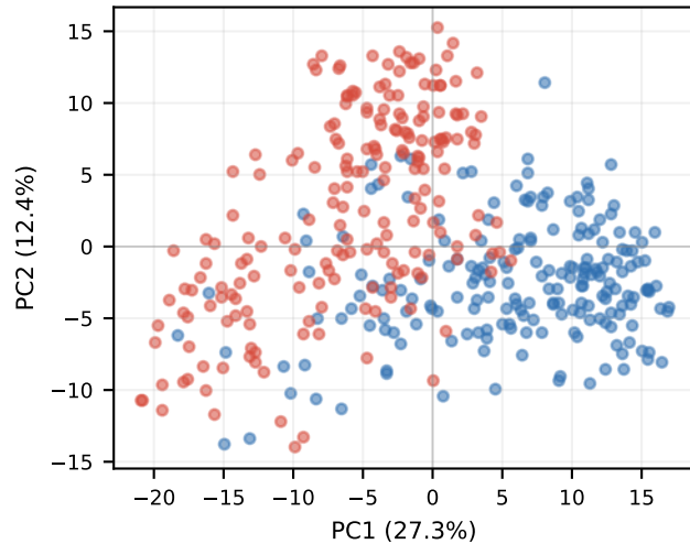
KD-NonChat Layer 6
