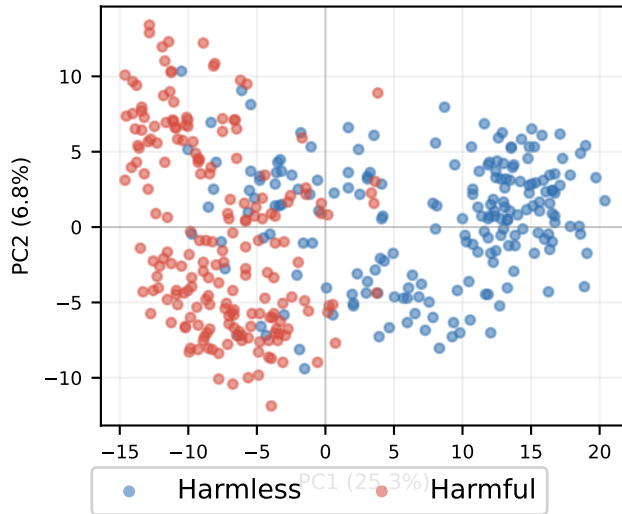
KD-Chat Layer 6
