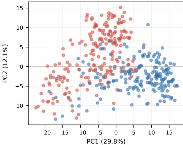
Base Layer 6
