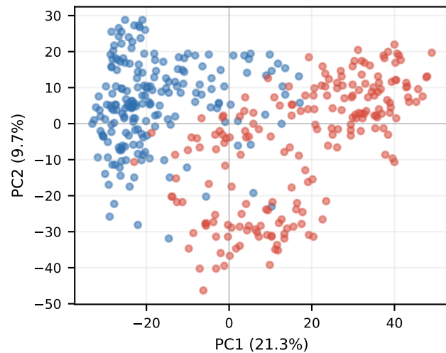
KD-NonChat Layer 8
