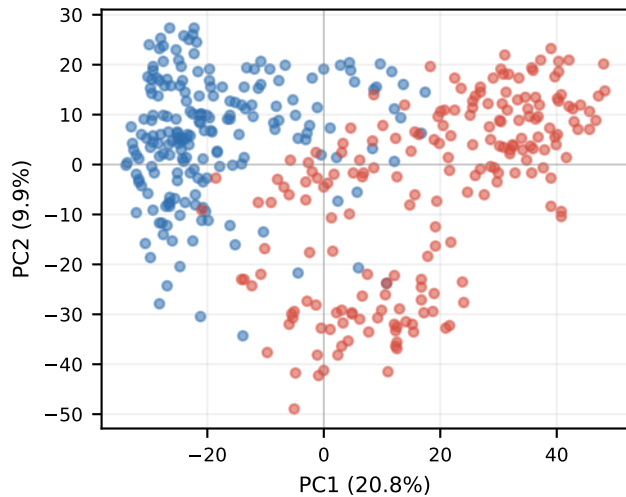
Base Layer 8
