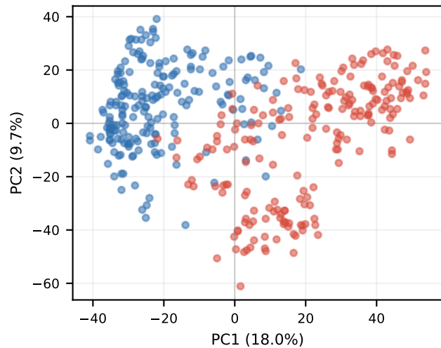
Base Layer 9
