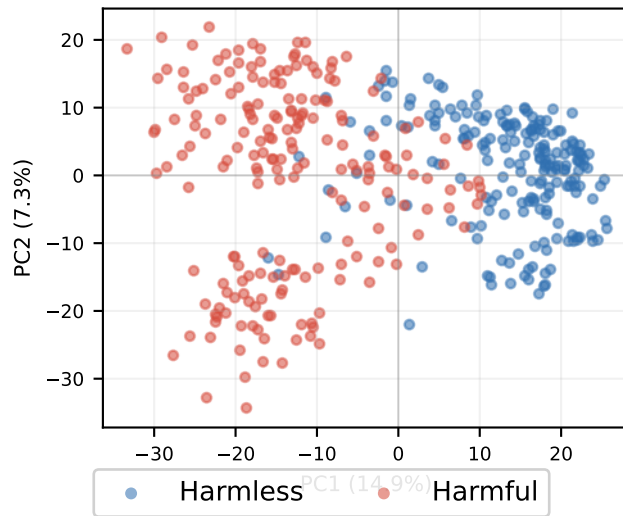
KD-Chat Layer 9
