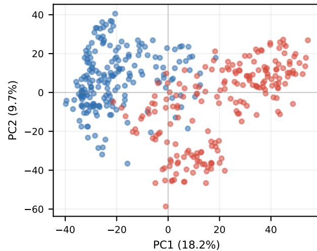
KD-NonChat Layer 9
