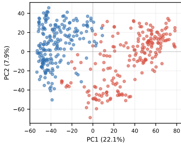
Base Layer 11
