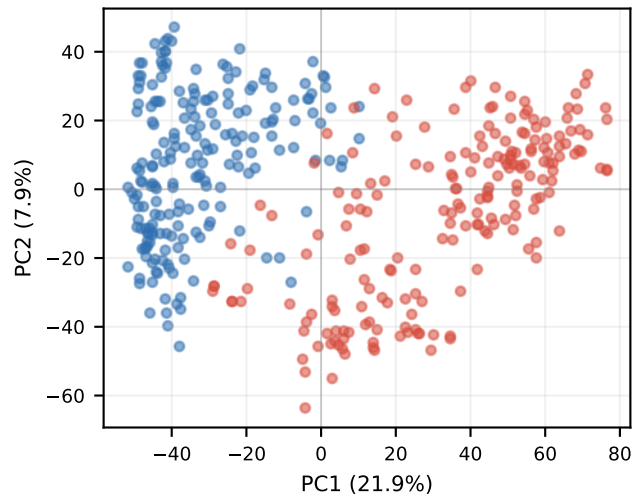
KD-NonChat Layer 11
