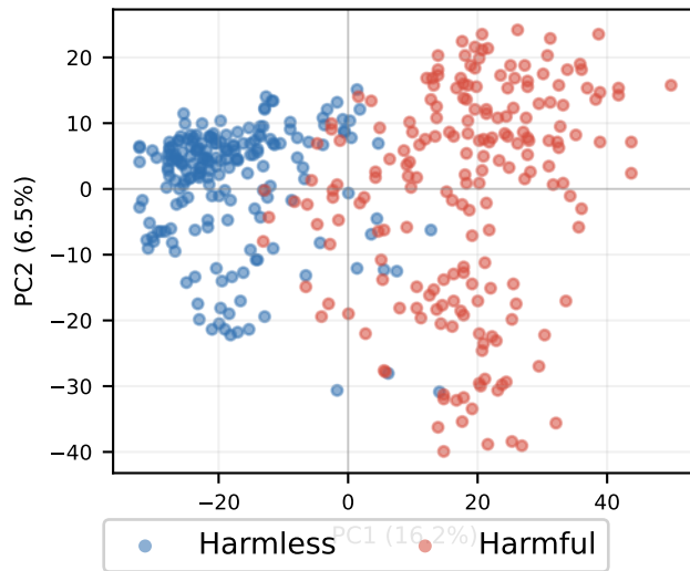
KD-Chat Layer 11
