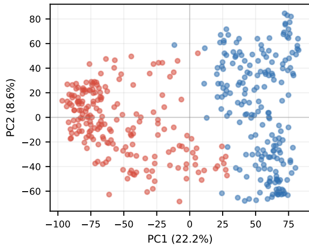
Base Layer 14
