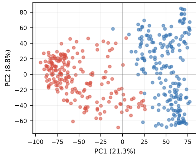
KD-NonChat Layer 14
