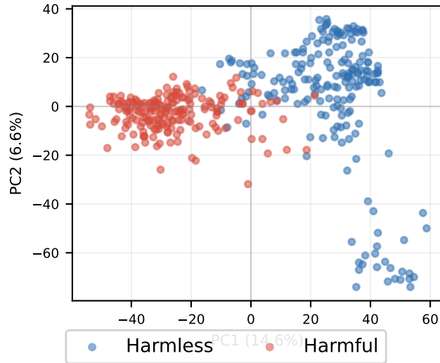
KD-Chat Layer 14
