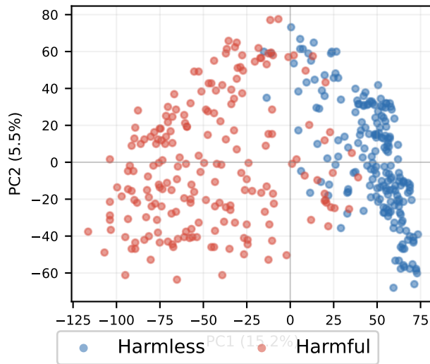
KD-Chat Layer 18
