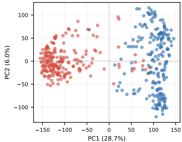
KD-NonChat Layer 18
