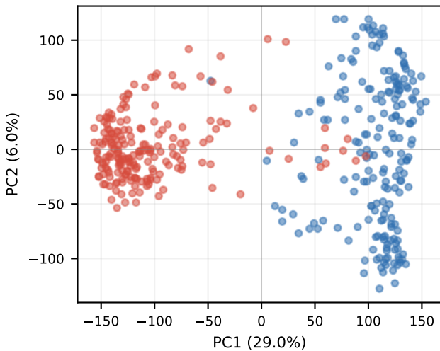
Base Layer 18
