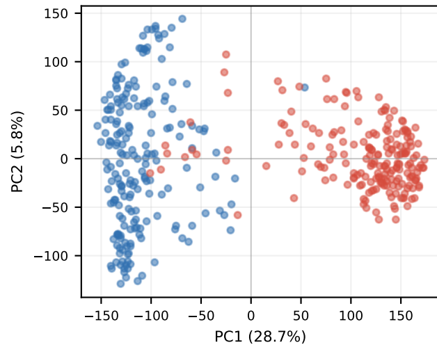
KD-NonChat Layer 19
