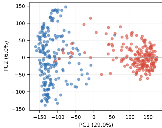
Base Layer 19
