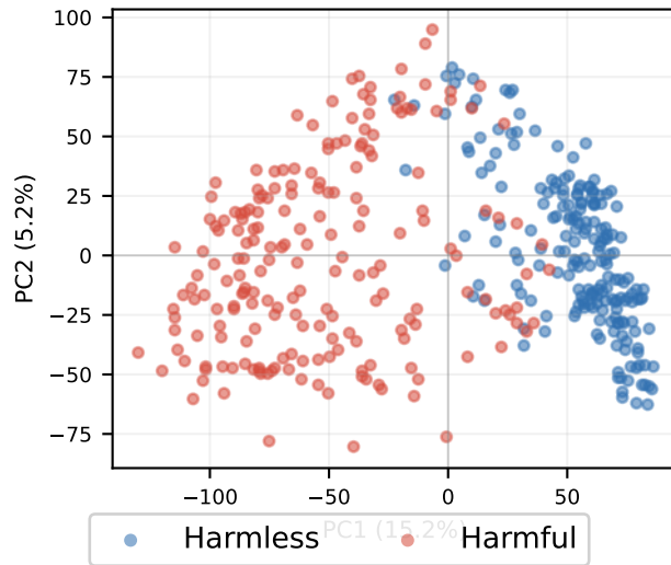
KD-Chat Layer 19
