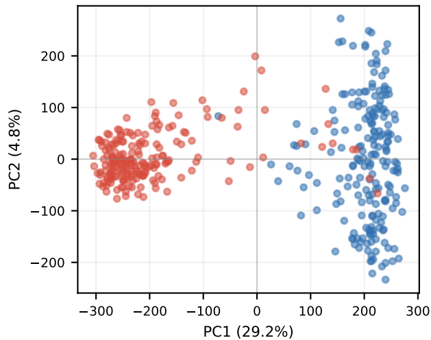
Base Layer 24
