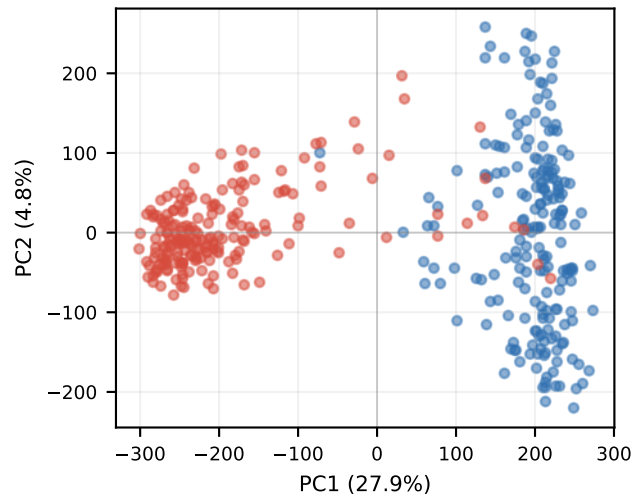
KD-NonChat Layer 24
