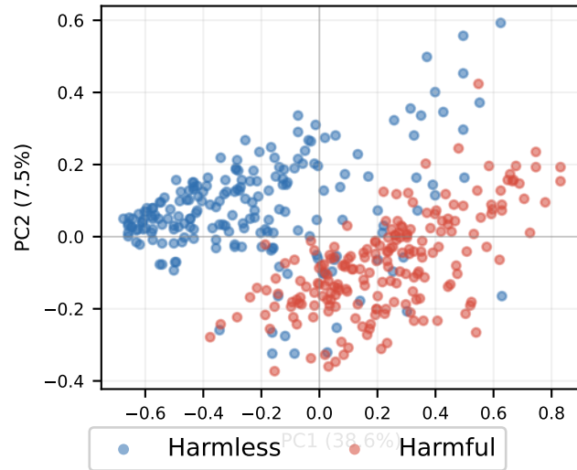
KD-NonChat Layer 2
