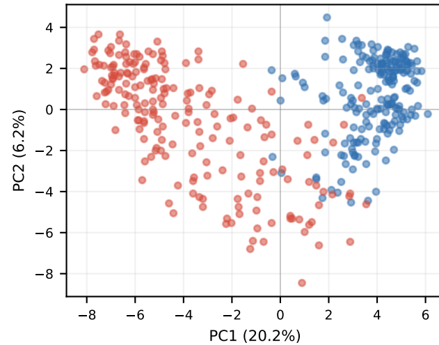
KD-Mix-C0.6 Layer 17
