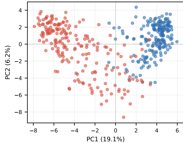
KD-Chat Layer 17
