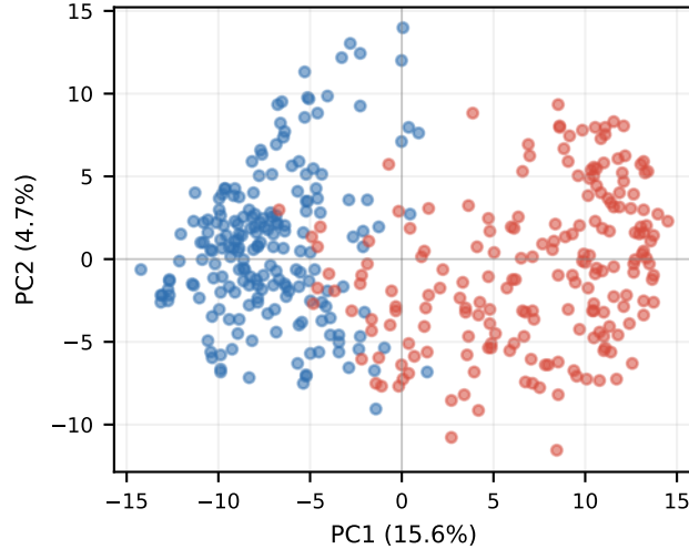
KD-Chat Layer 23
