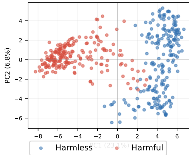
KD-NonChat Layer 16
