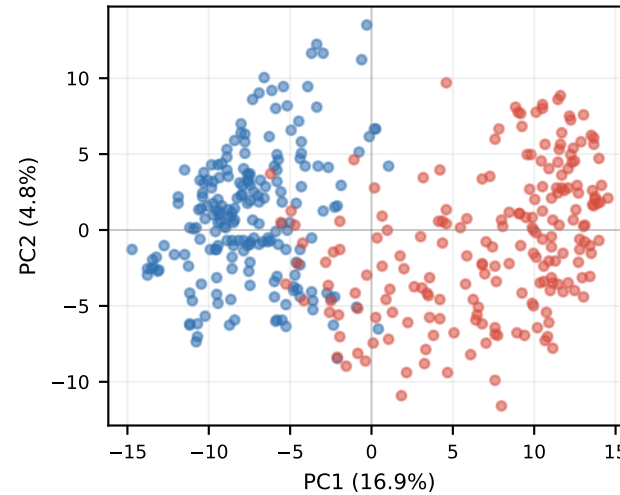
KD-Mix Layer 23
