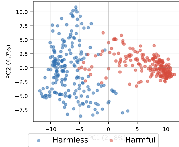
KD-NonChat Layer 21
