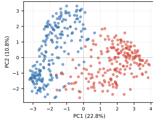
KD-Mix Layer 11
