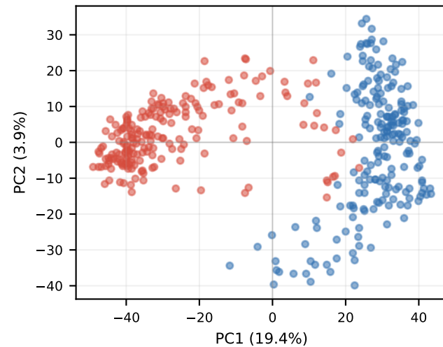
Base Layer 27
