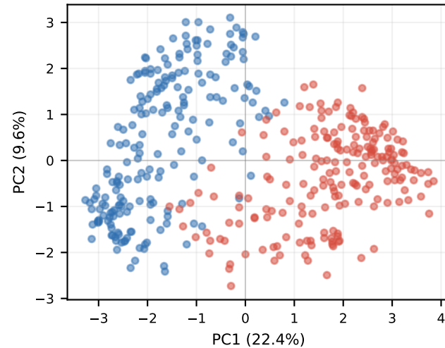
KD-Mix-C0.6 Layer 11
