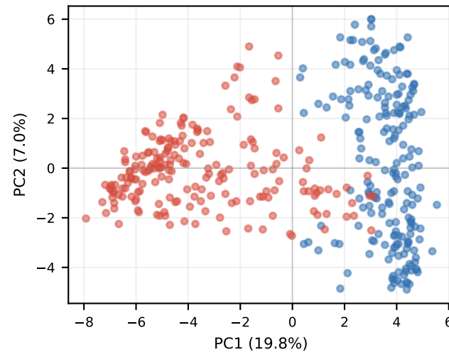
KD-Mix Layer 16
