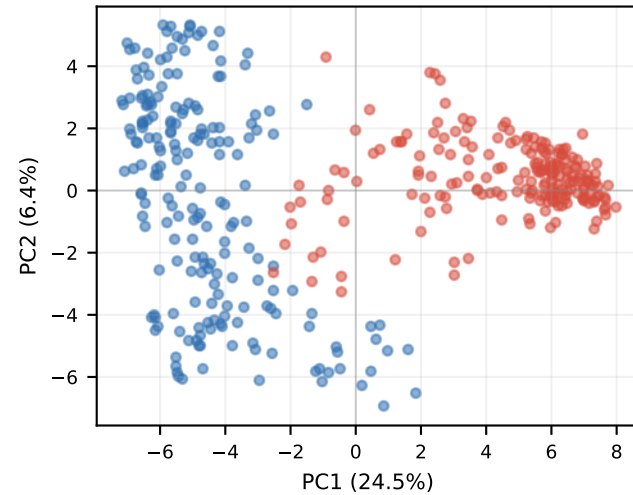
Base Layer 17
