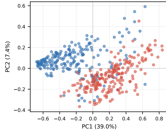
KD-Mix Layer 2
