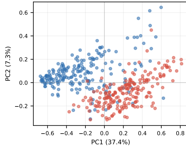
KD-Mix-C0.6 Layer 2
