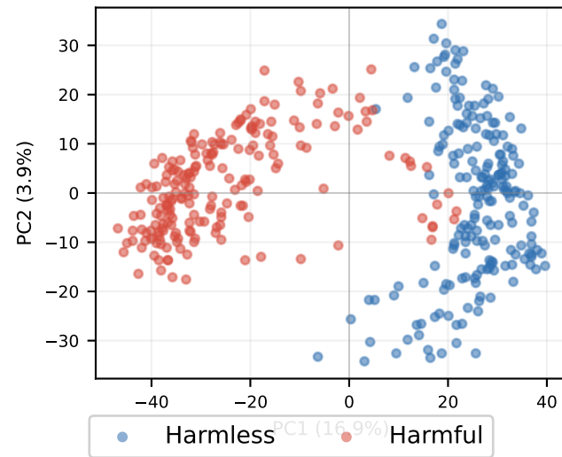
KD-NonChat Layer 27
