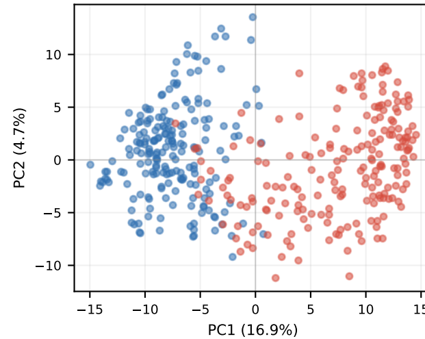
KD-Mix-C0.6 Layer 23
