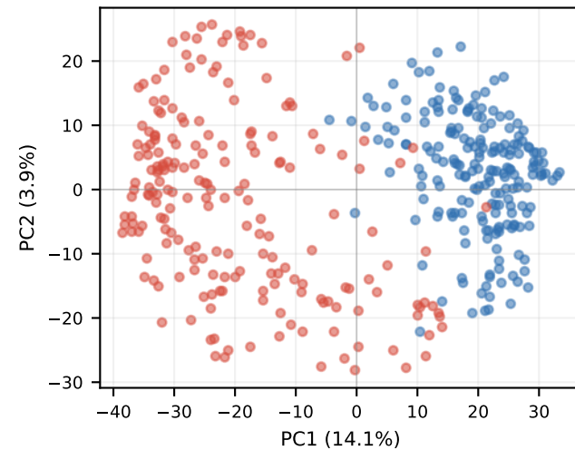
KD-Mix-C0.6 Layer 27
