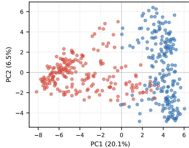
KD-Mix Layer 17
