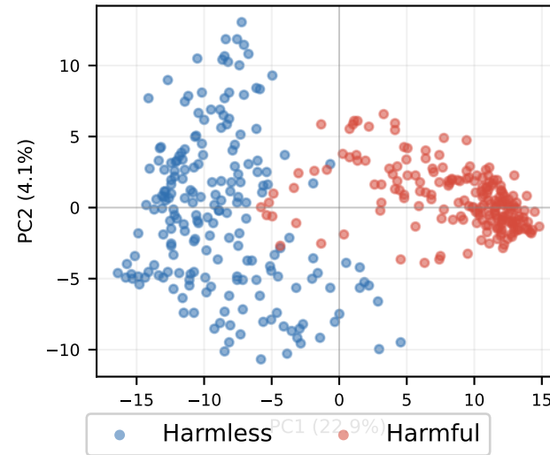
KD-NonChat Layer 23
