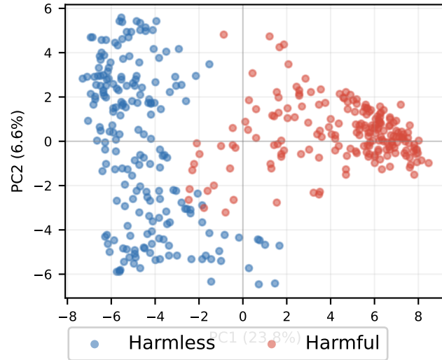
KD-NonChat Layer 17
