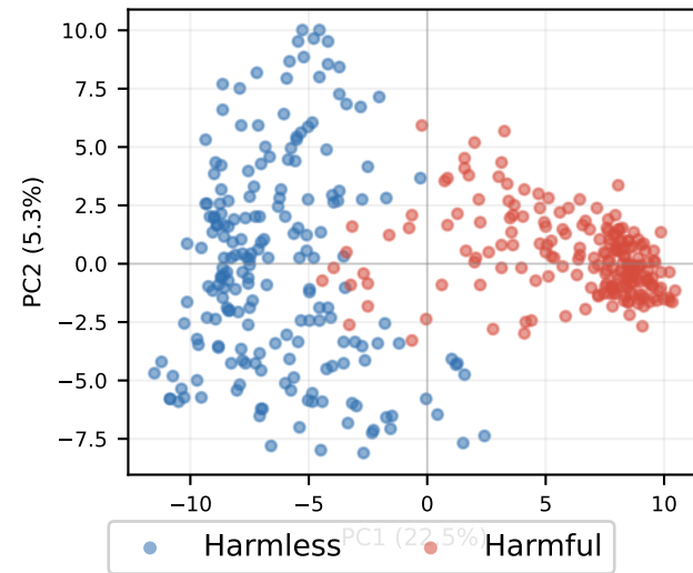
KD-NonChat Layer 20
