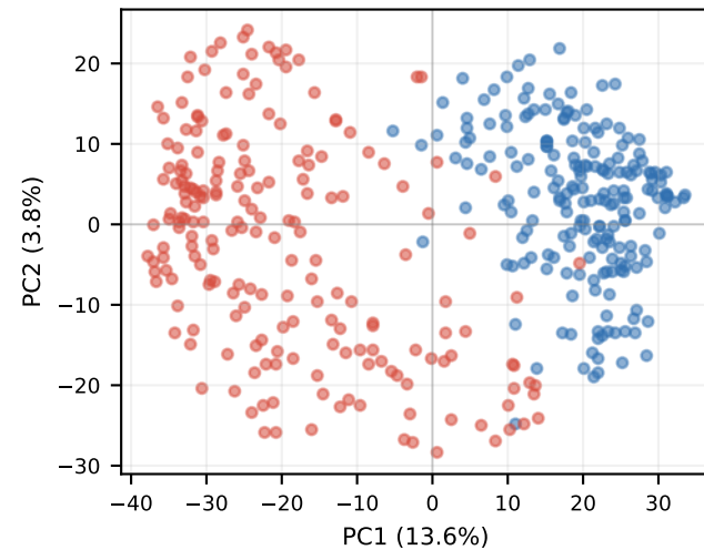
KD-Mix Layer 27
