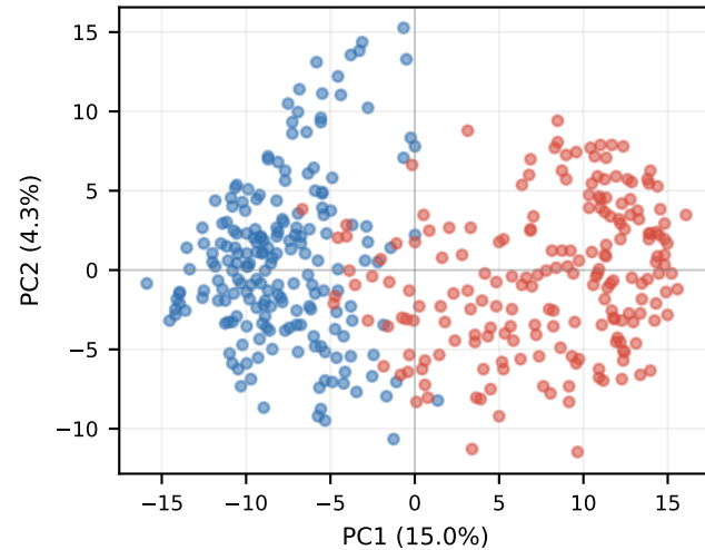
KD-Chat Layer 24
