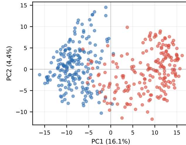
KD-Mix Layer 24
