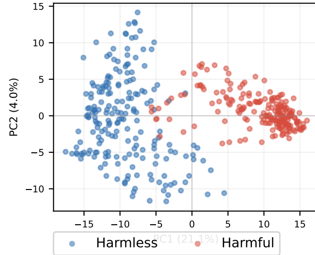
KD-NonChat Layer 24
