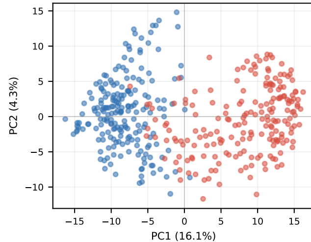
KD-Mix-C0.6 Layer 24
