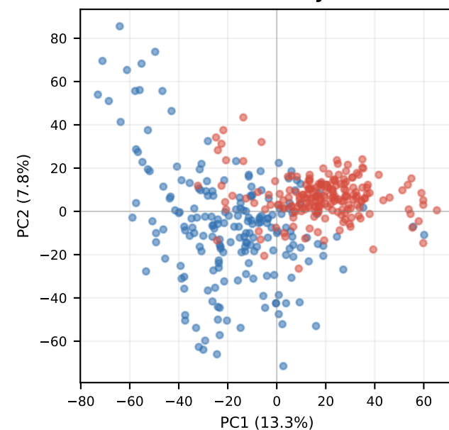
KD-Chat Qwen-2.5-3B layer 35
