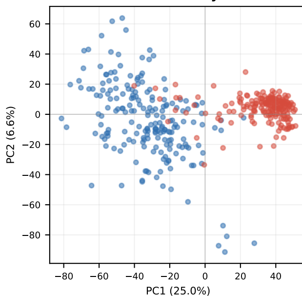
KD-NonChat Qwen-2.5-3B layer 35
