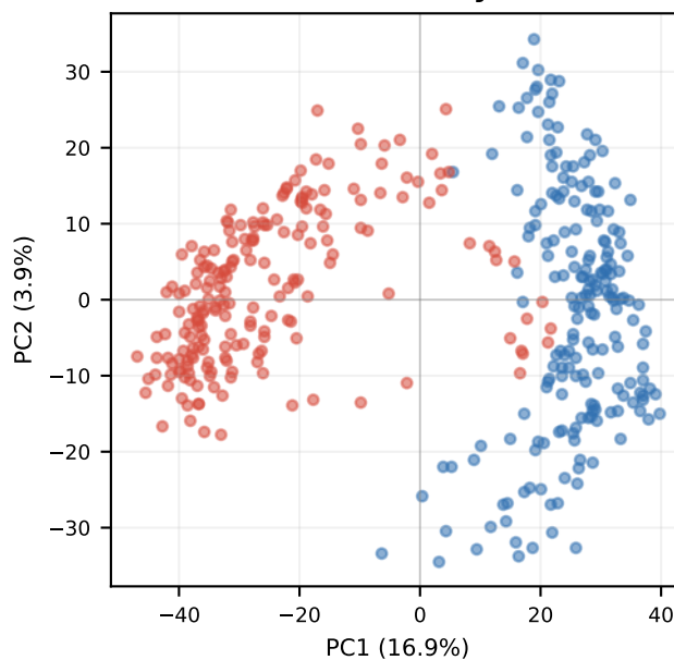
KD-NonChat Gemma-2-2B layer 25
