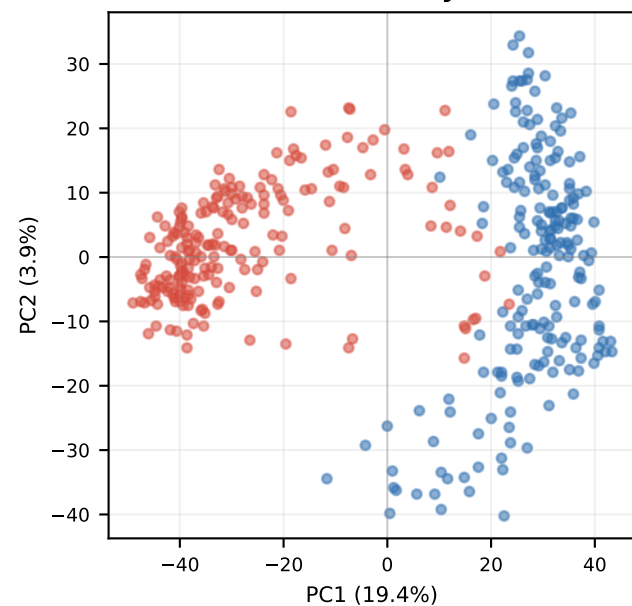
Base Gemma-2-2B layer 25
