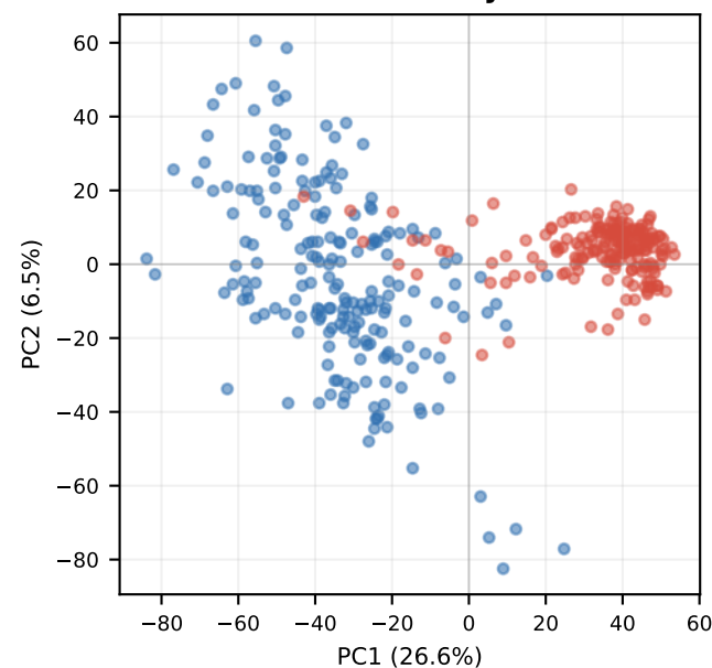
Base Qwen-2.5-3B layer 35
