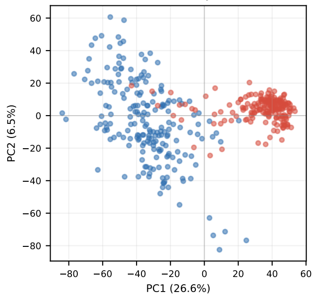
Base Gemma-2-2B layer 25
