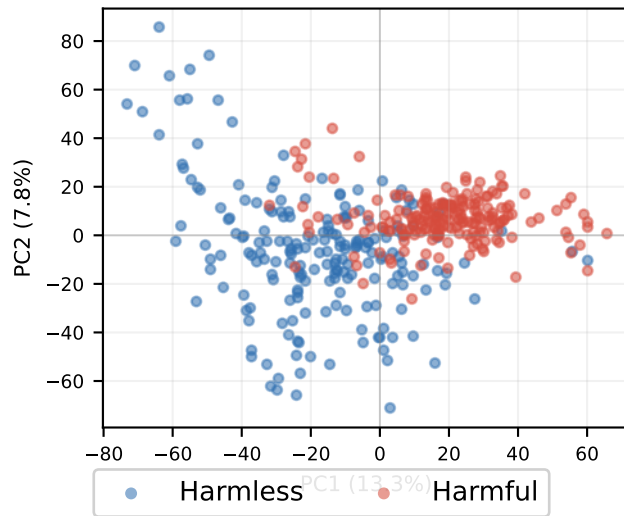
KD-Chat Layer 25
