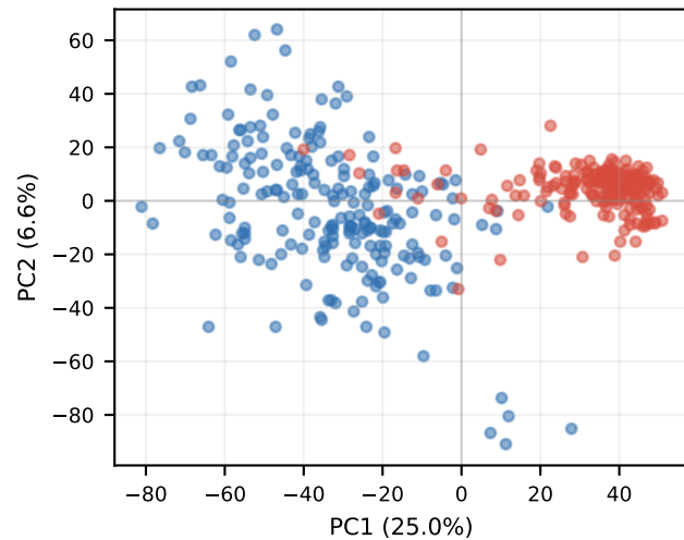
KD-NonChat Layer 25
