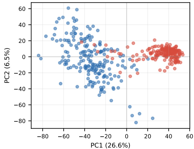
Base Layer 25
