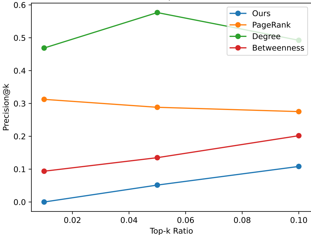
CiteSeer Top-k Precision
