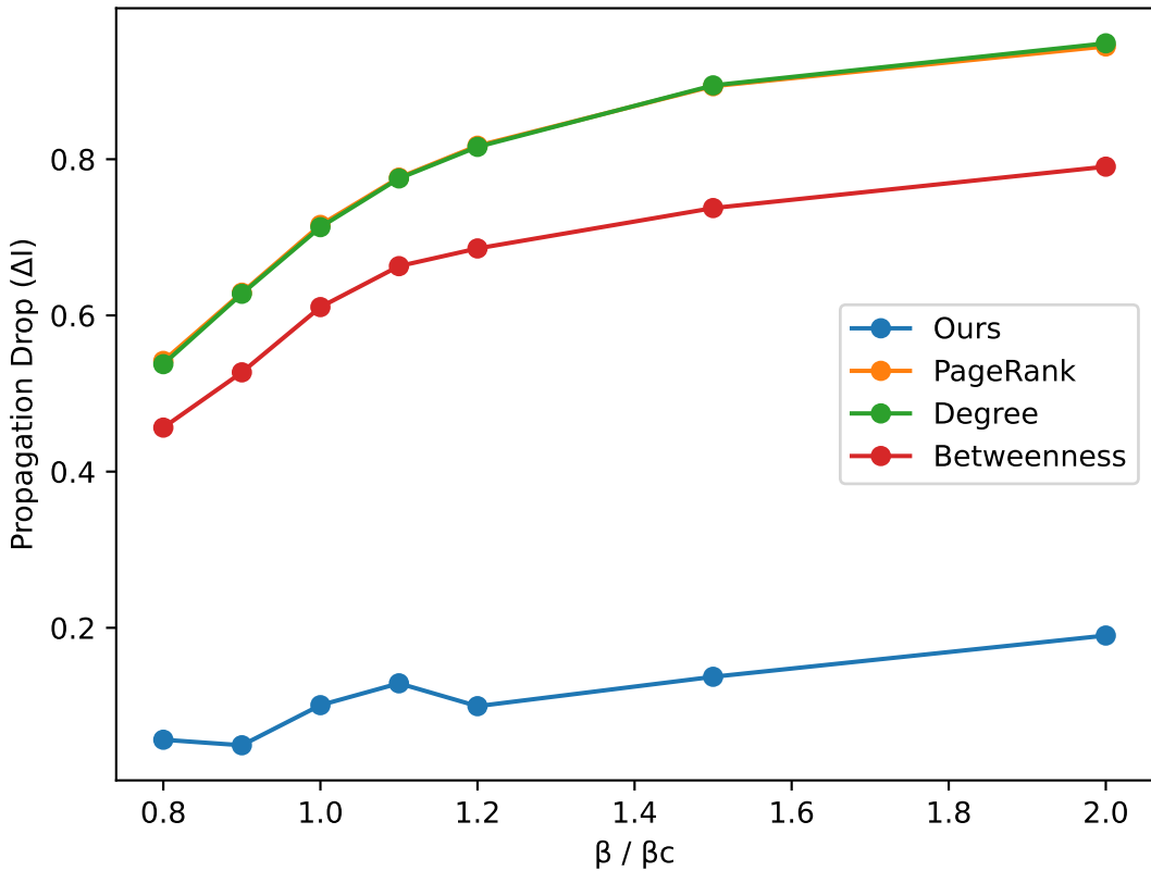
CiteSeer Robustness
