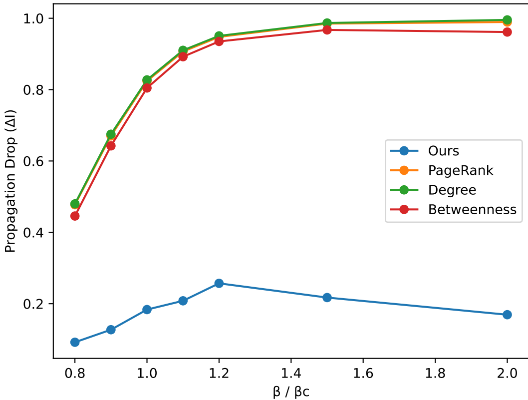
PubMed Robustness
