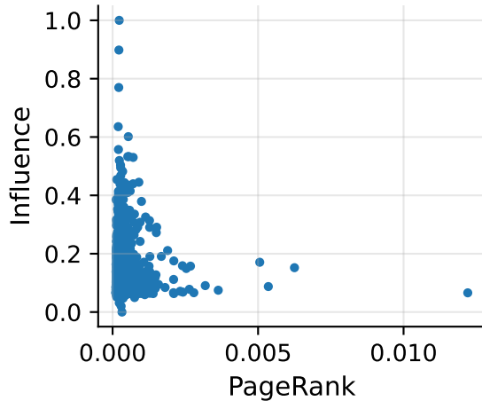
PageRank \rho=0.05
