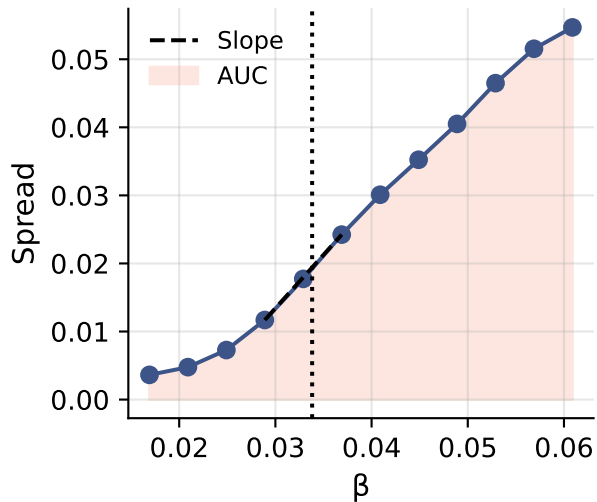
(d) Slope and AUC Illustration
