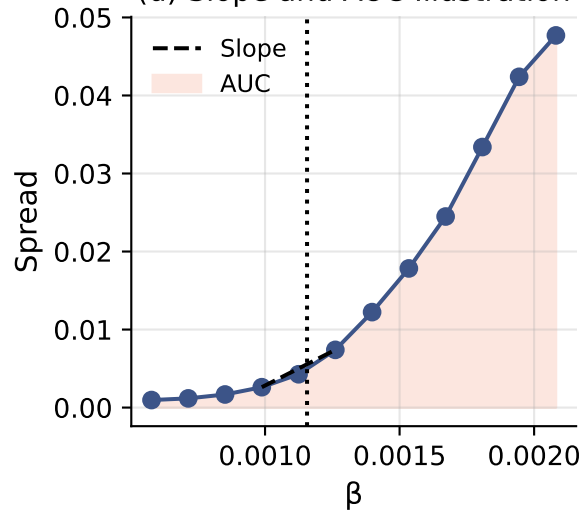
(d) Slope and AUC Illustration
