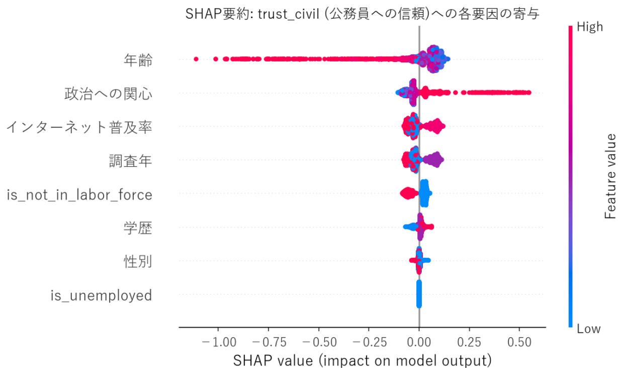
図1 SHAP 要約プロット：公務員への信頼に対する各説明変数の寄与（Random Forest, ISSP 日本データ）
