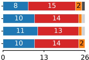
Devstral
