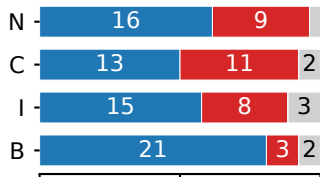
GPT-5.5 Low
