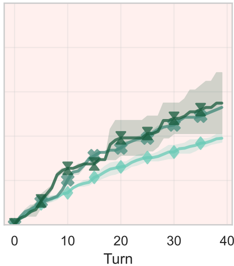
Item ASR
