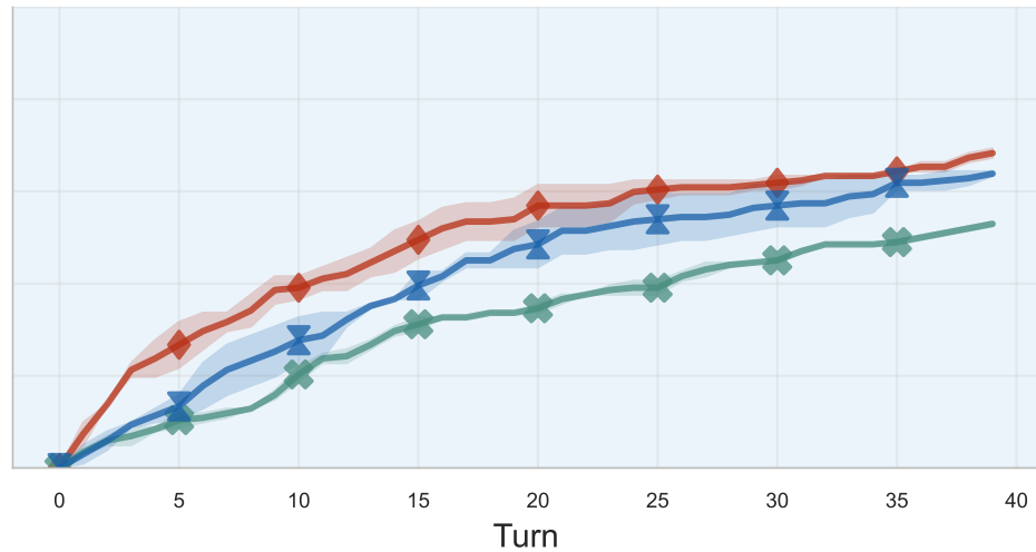
Item ASR
