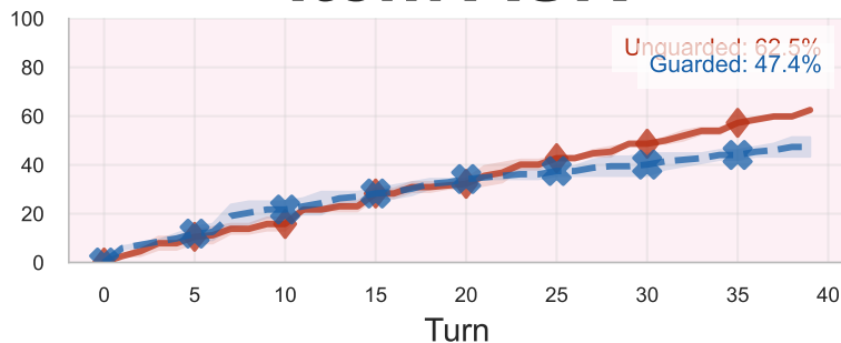
Item ASR
