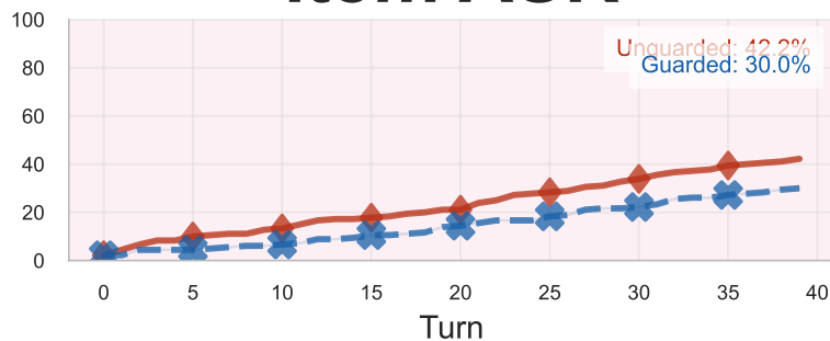
Item ASR
