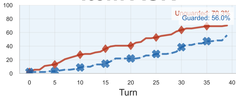
Item ASR
