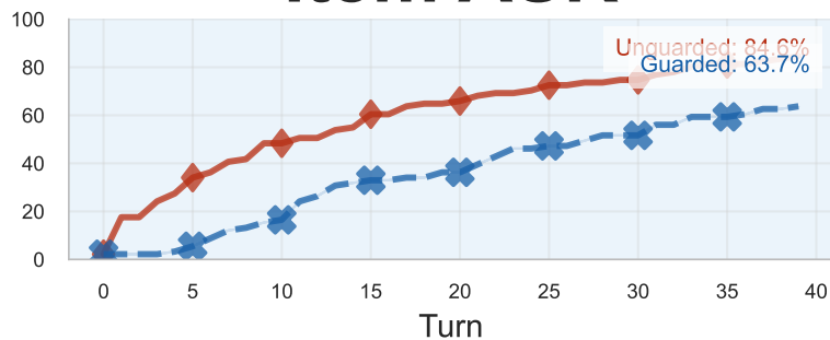
Item ASR
