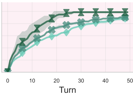
Item ASR
