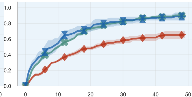
Item ASR
