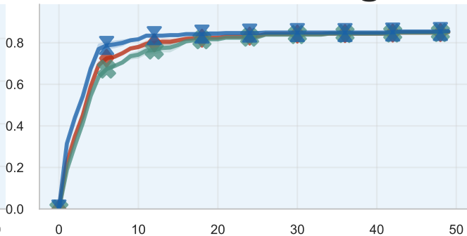
Edge FPR
