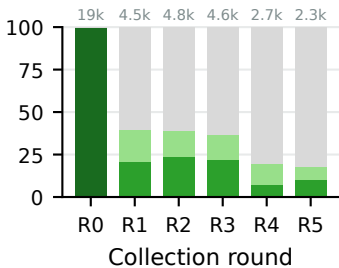
HiL-IDQL+Mulligan
