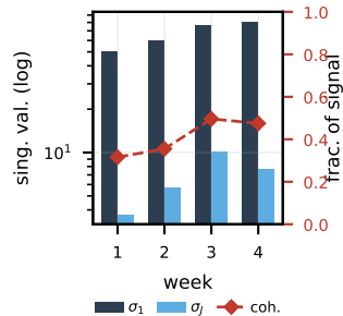
(d) Obs. geometry
