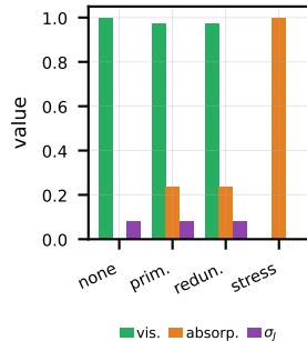
(d) Exp: bg. stress
