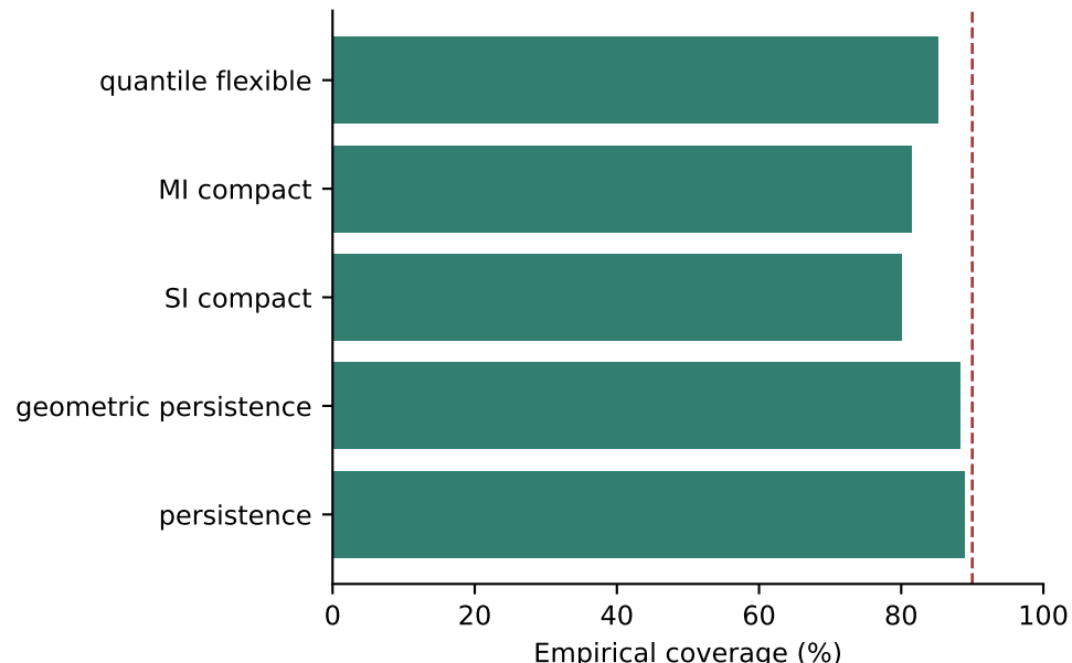
Colorado: nominal 90% intervals
