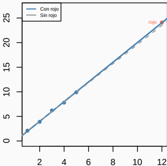
A: Leverage alto, Cook bajo
