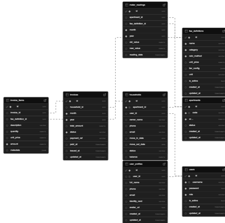
Hình 3.1: Biểu đồ quan hệ thực thể ERD
