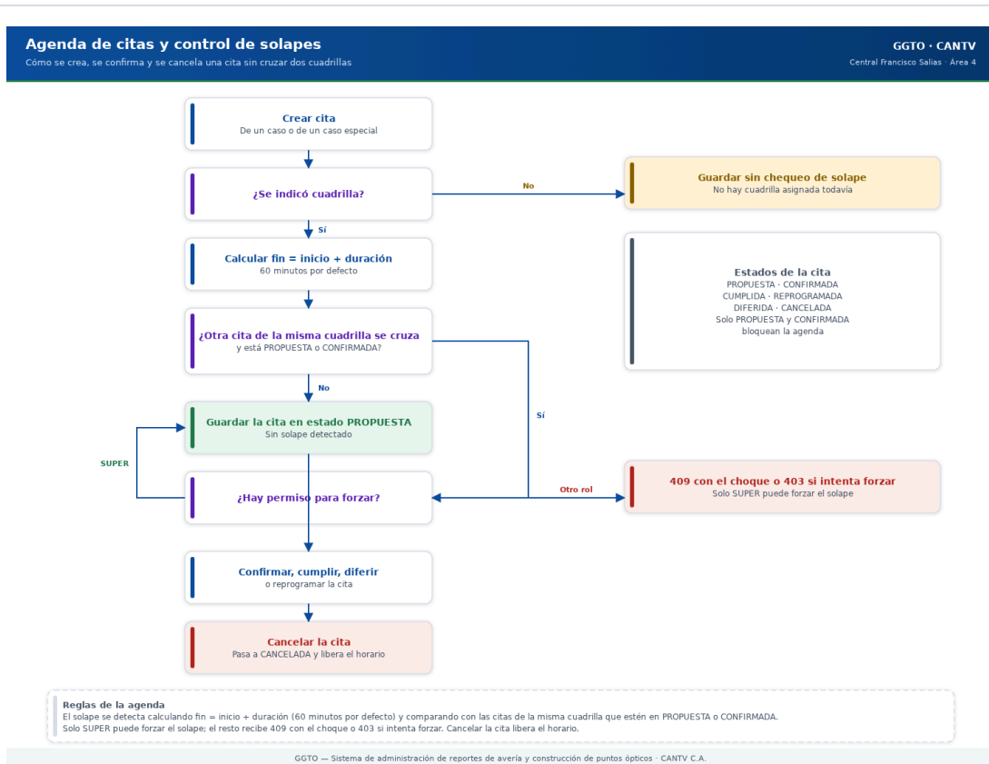
Figura 2 · agenda-citas.png
