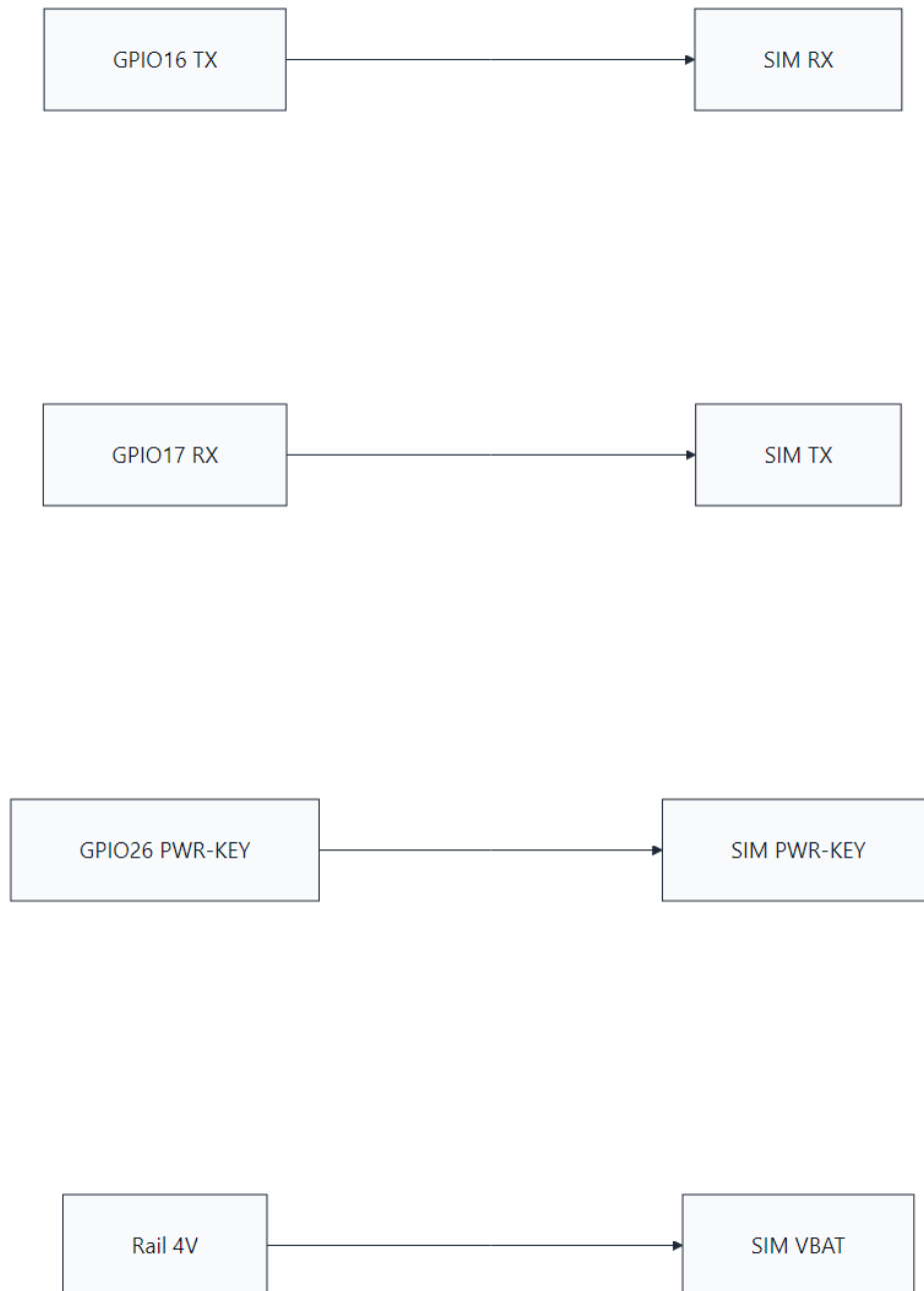
Hình 4.2: Sơ đồ kết nối giữa ESP32-S3 và modem SIM7600CE-T qua UART
