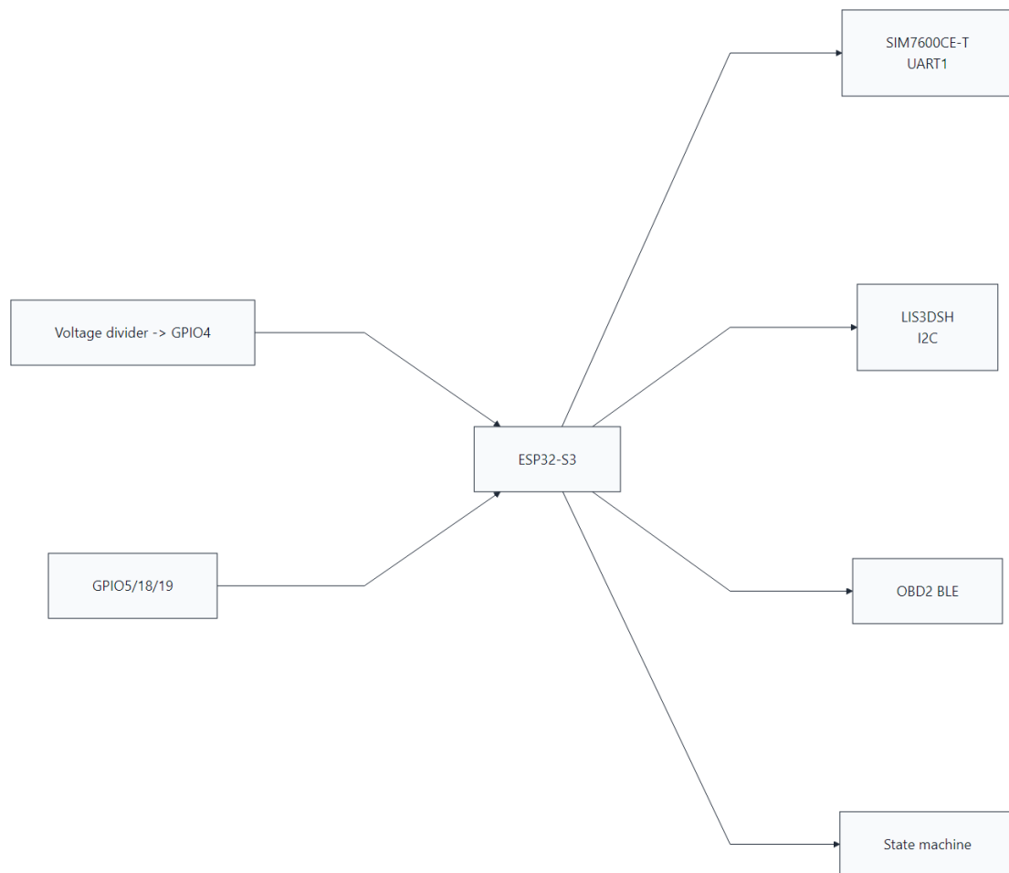
Hình 4.5: Sơ đồ đấu nối tổng thể giữa ESP32-S3 và các khối phần cứng tích hợp
