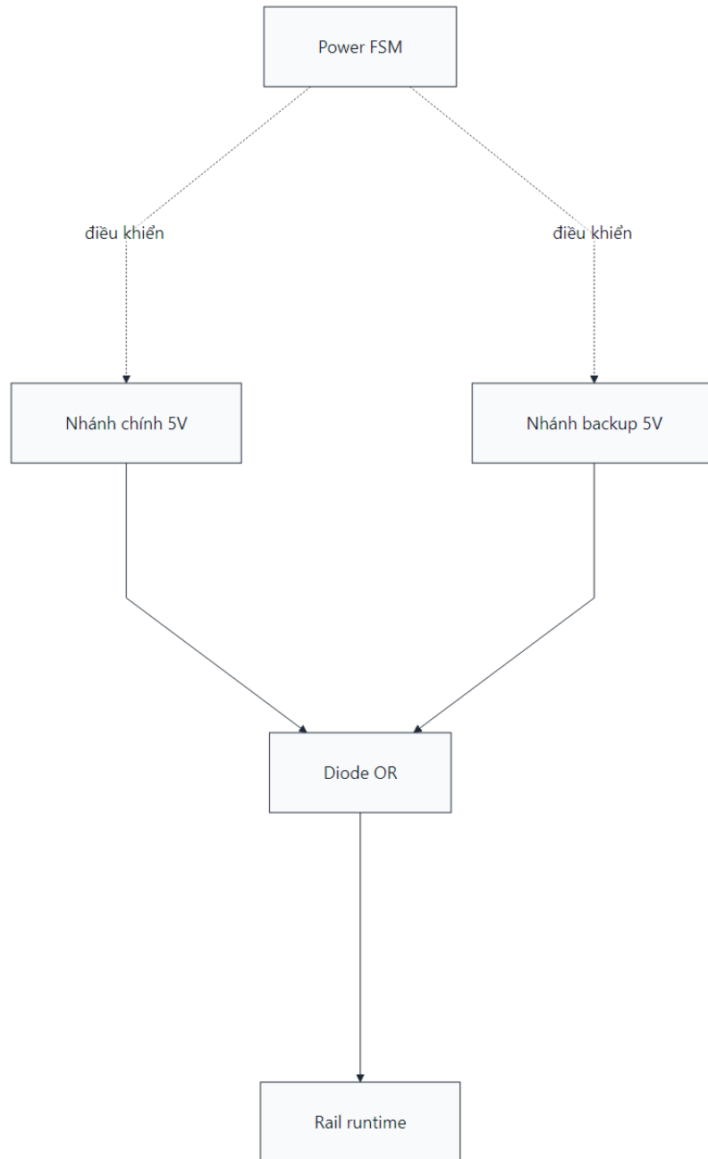
Hình 4.6a: Kiến trúc power path giữa nguồn xe và pin dự phòng
