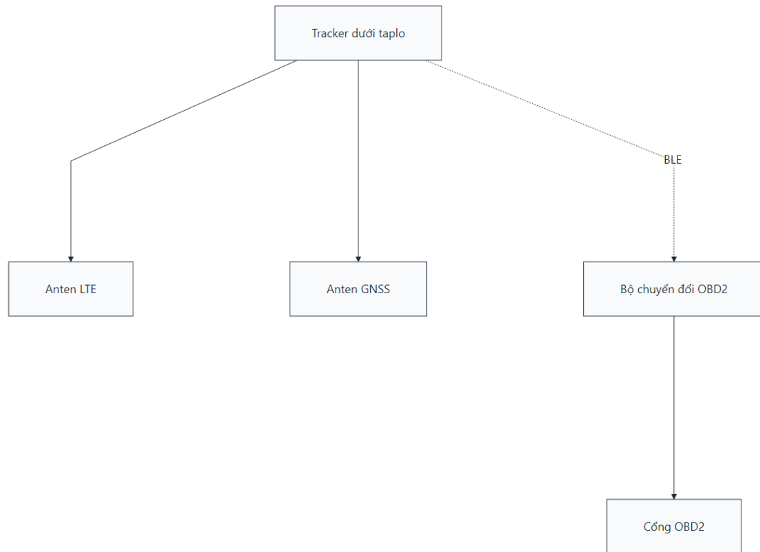
Hình 4.15: Minh họa lắp đặt thiết bị tracker trong xe và đi dây
