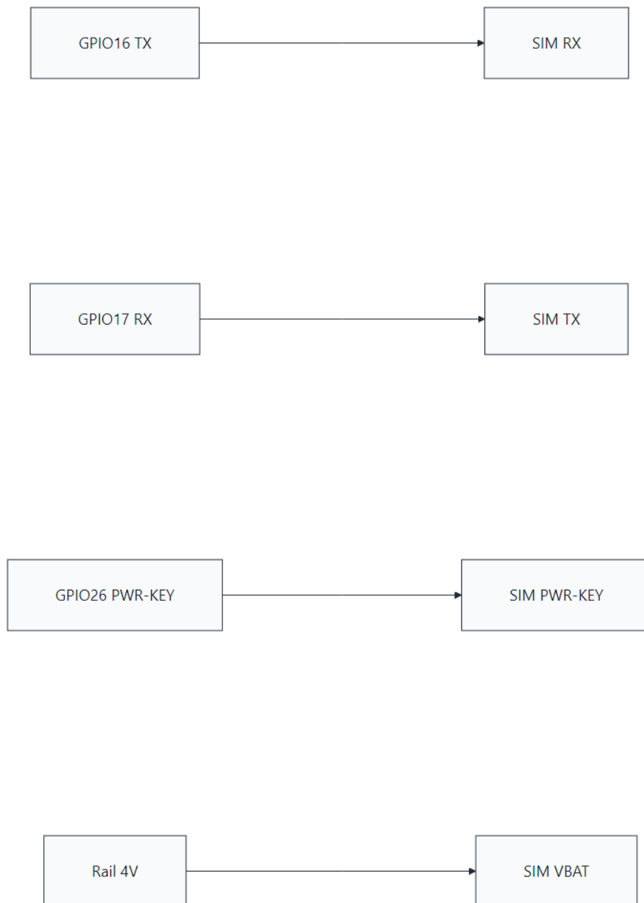
Hình 4.2a: Sơ đồ chân kết nối SIM7600CE-T với ESP32-S3
