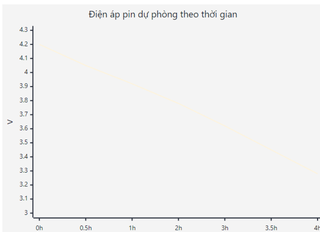
Hình 4.33: Đồ thị điện áp pin dự phòng theo thời gian theo baseline 18650 trong kịch bản tracking liên tục
