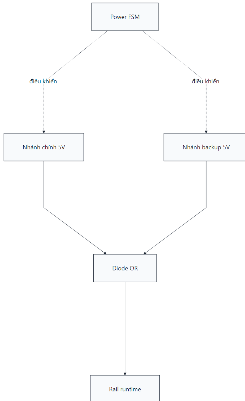
Hình 4.9: Sơ đồ power path runtime giữa nhánh chính và nhánh backup
